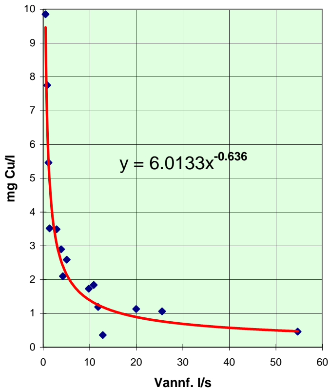
Figur 2. Sammenhengen mellom kobberkonsentrasjoner og vannføring ved St.1 Måledam for samlet avrenning fra Kjøli gruve.
