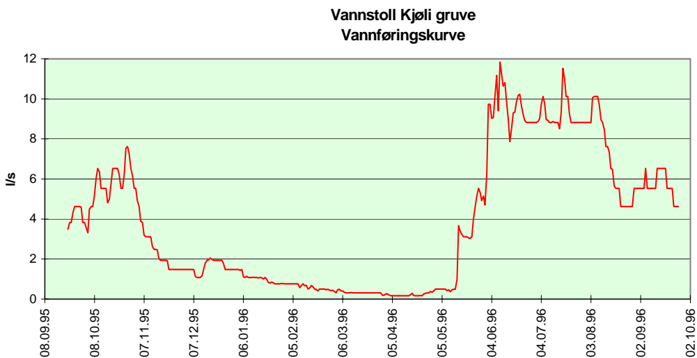
Figur 5. Døgnmiddelvannføeringer ved st.2 Gruvevann ved utløp vannstoll Kjøli gruve.
