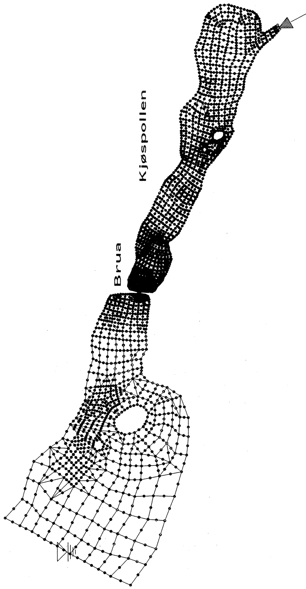
Figur 4.1. Bottopografien i Kjøsapollen er lagt inn i den numeriske modellen SMR/RMA2 som eit nettverk eller "grid" som er konstruert i følgje endelig-element metoden. Modellen reknar numeriske løysingar for dynamikken (strøm, vannstand) i alle knutepunkta.
