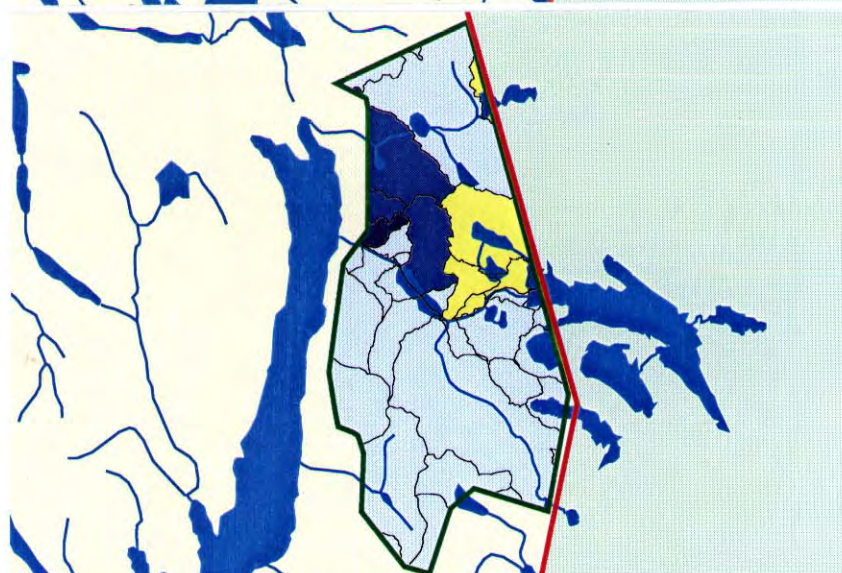
Figur 4. Femundsmarka nasjonalpark: Tålegrenser for tilførsler av syre ved bruk av ANC_{var} og vannprøver i tabell 2. Overskridelse av tålegrensen for tilførsler av svovel og nitrogen er basert på dagens S-deposisjon (1990) og scenarier for S-deposisjon i år 2010 og dagens N-avrenning.
