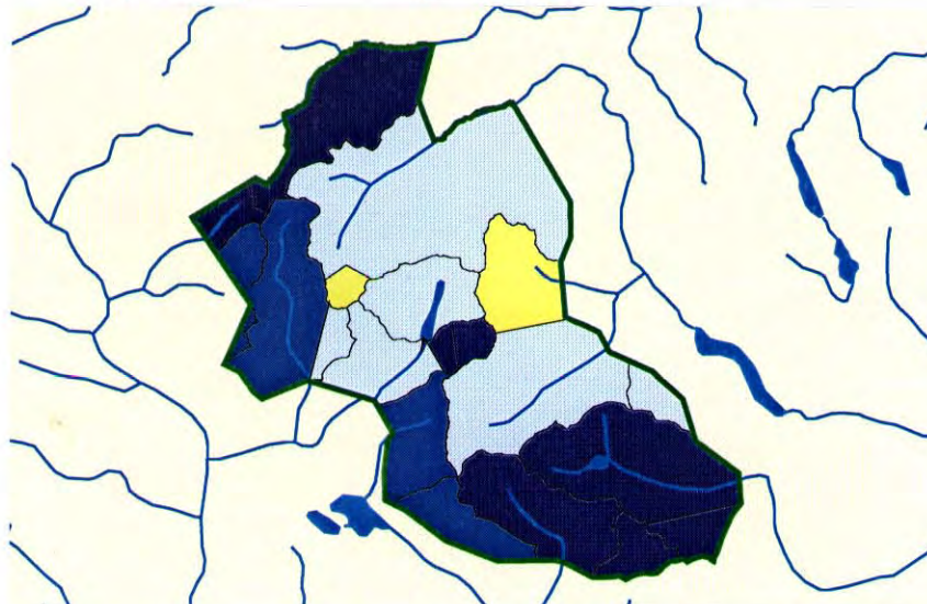
Figur 5. Rondane nasjonalpark: Tålegrenser for tilførsler av syre ved bruk av ANC var og vannprøver i tabell 3. Overskridelse av tålegrensen for tilførsler av svovel og nitrogen er basert på dagens S-deposisjon (1990) og scenarier for S-deposisjon i år 2010 og dagens N-avrenning.
