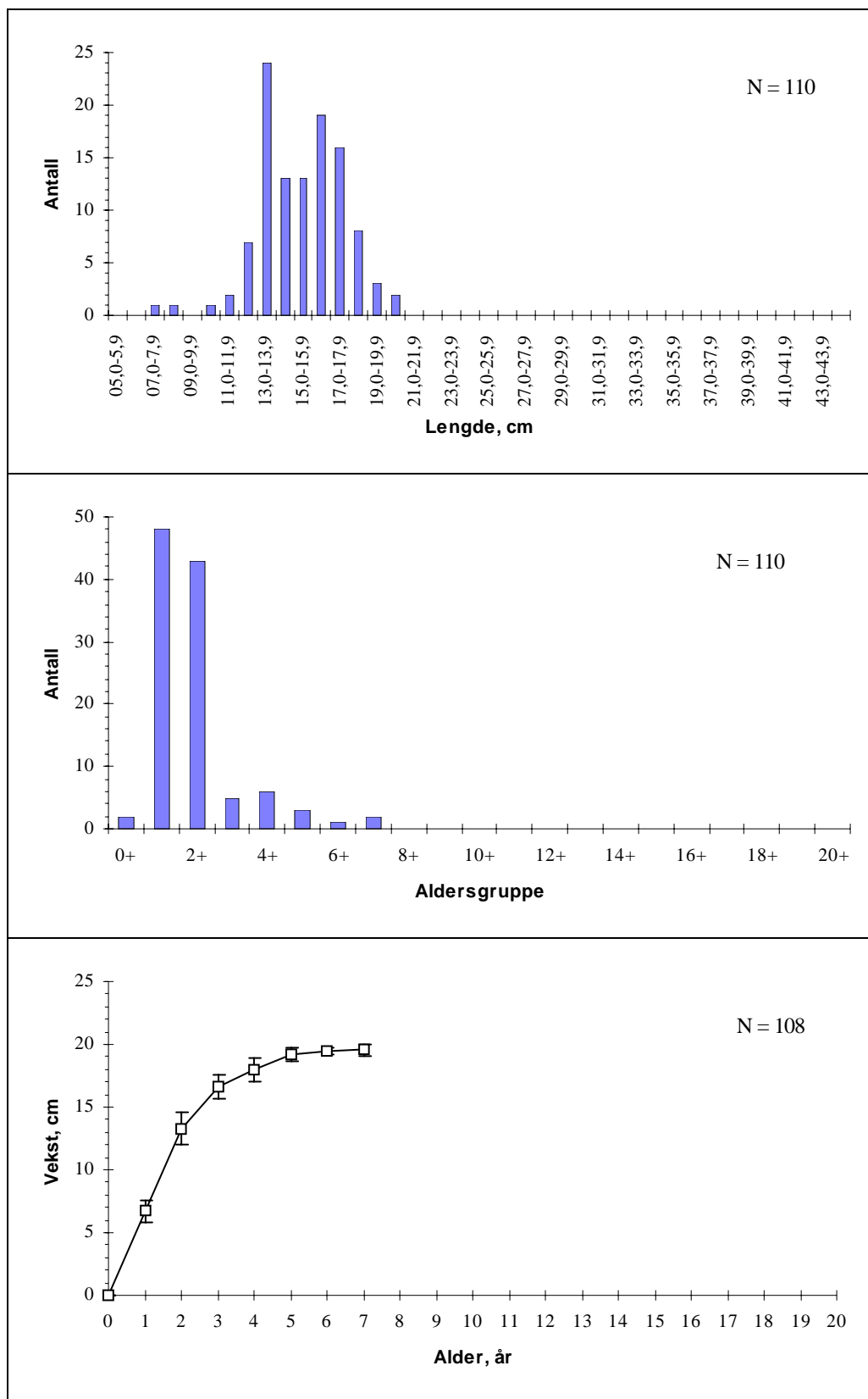
Figur 17. Lengdefordeling, aldersfordeling og tilbakeregnet vekst for tryte i Molandsvatn i 1985.
