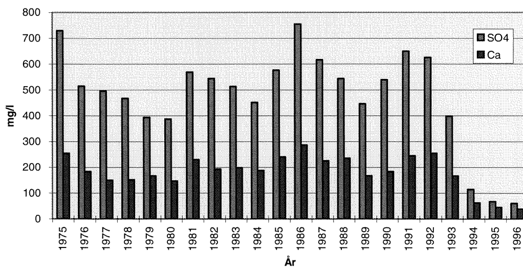
Figur 9. Tidsveiede middelverdier for kalsium og sulfat ved overløp av slamdam, Hjerkin.
