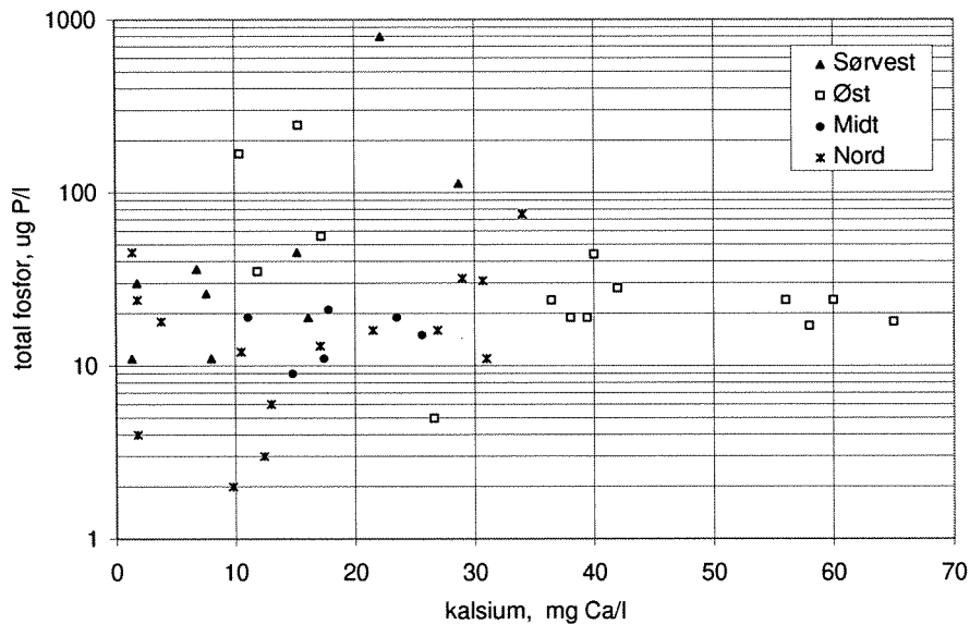
Figur 2. Fordeling av innsjøene langs fosfor- og kalsium-gradienten.
