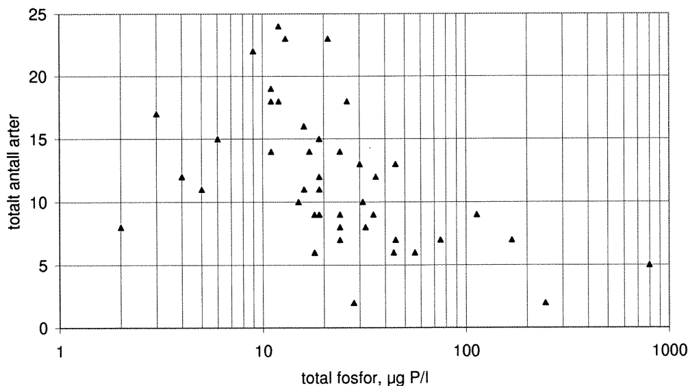
Figur 6. Variasjon av total antall arter (karplanter + kransalger) langs trofigradienten for alle 44 innsjøene.
