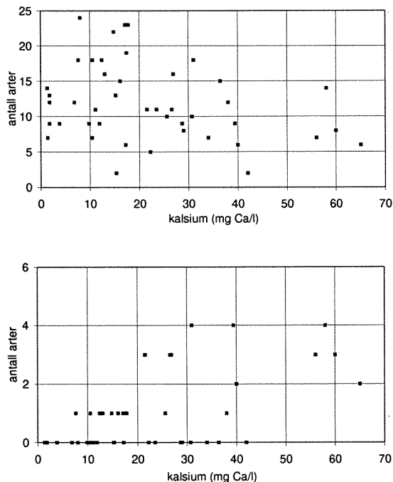
Figur 5. Variasjon i Totalt antall arter (øverst) og Antall kransalger innenfor slekta Chara (nederst) langs kalsiumgradienten for de 44 innsjøene.
