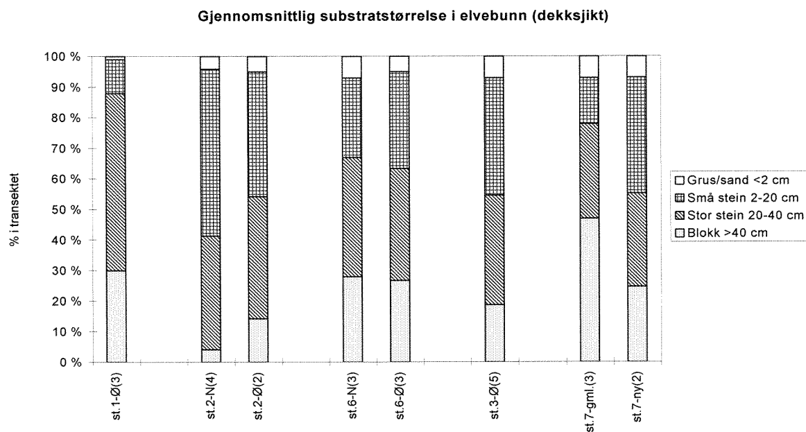
Figur 3. Gjennomsnittlig substratstørrelse i øvre (Ø) og nedre (N) transect. Antall observasjoner i parentes. Atnavassdraget 1990-95.
