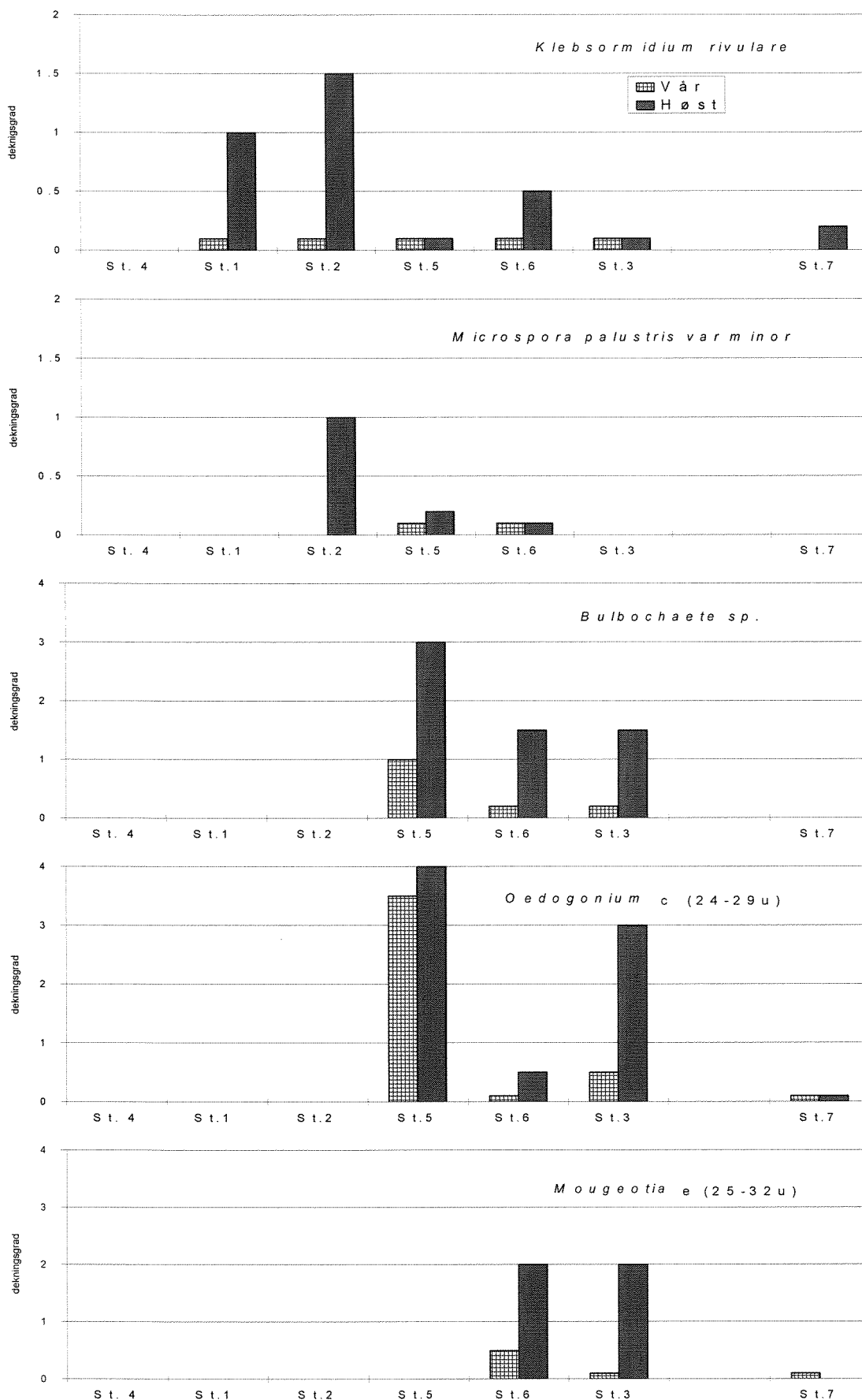
Figur 7A. Karakterarter av trådformede grønnealger, midlere dekningsgrad , basert på subjektiv mengdevurdering i årene 1989-95. Øvre del av Atnavassdraget. NB! Figurene har ulik skala.
