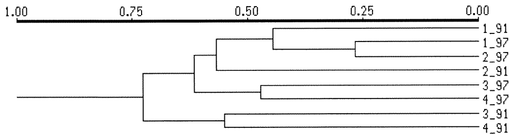
Figur 21. Klusteranalyser av stasjoner i 1989 (data fra Helland og Rygg 199) og 1997. Stasjonsnummer og årstall er angitt i loddrett tallkode (for data fra 1989 er publiseringsår angitt). Skalaen langs den vannrette aksene viser grad av ulikhet. Lavest tall viser størst likhetsgrad.
