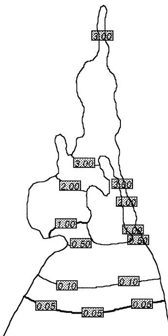
Figur 7. Fordeling av MEG angitt i mg/l i Kvaliosen etter 1 døgn etter utslippet. MEG-konsentrasjonene gjelder for innlagringssjiktet som er antatt å være gjennomsnittlig 1 meter tykt over hele området.
