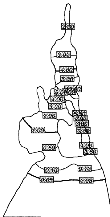
Figur 6. Fordeling av MEG angitt i mg/l i Kvaliosen etter 72 timer, det vil si når utslippet er stanset. MEG-konsentrasjonene gjelder for innlagringssjiktet som er antatt å være gjennomsnittlig 1 meter tykt over hele området.
