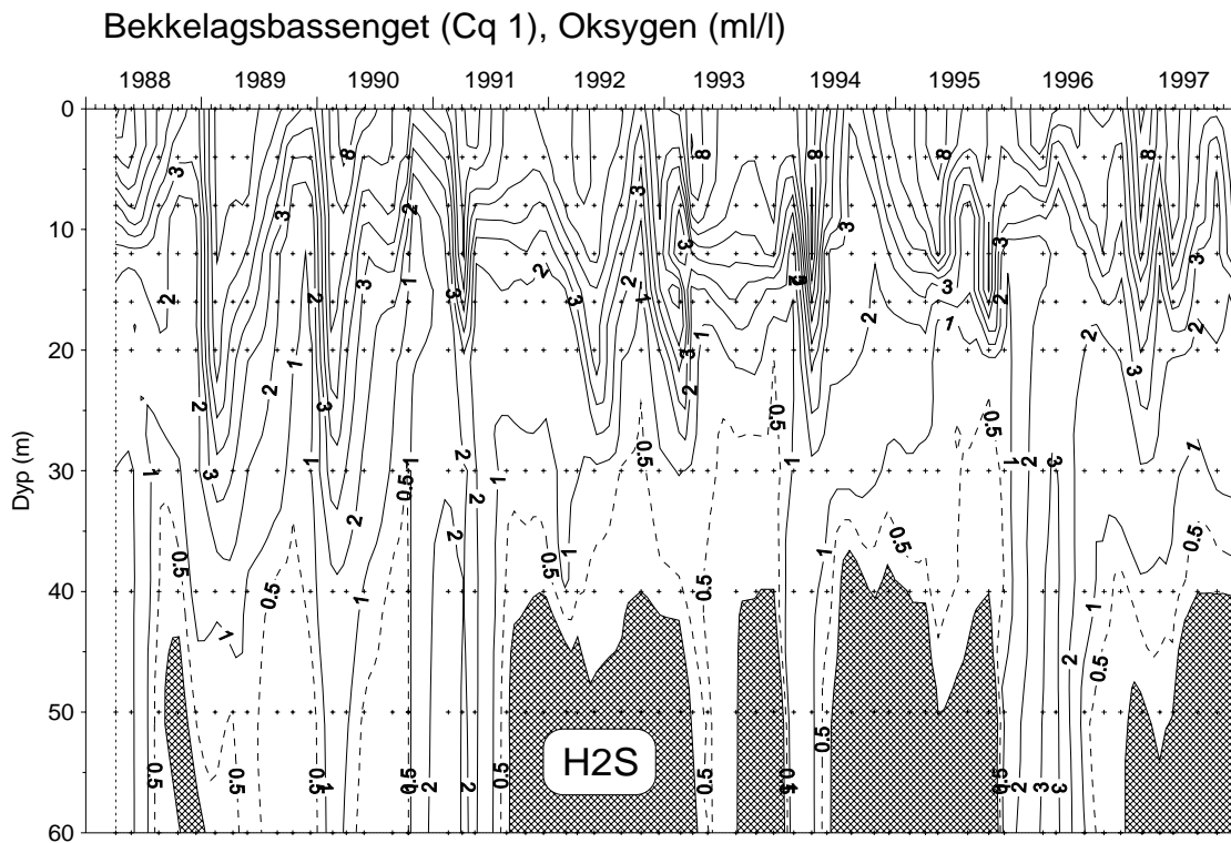
Figur 17. Oksygen/hydrogensulfid (ml/l) i Bekkelagsbassenget (Cq 1) 1988-1997.
