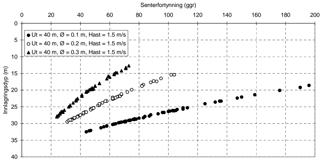
Figur 9. Innlagringsdyp (m) og senterfortynning (ggr) ved utslippsdyp 40 m, hullhastighet 1.5 m/s og hulldiametere 0.1, 0.2 og 0.3 m.
