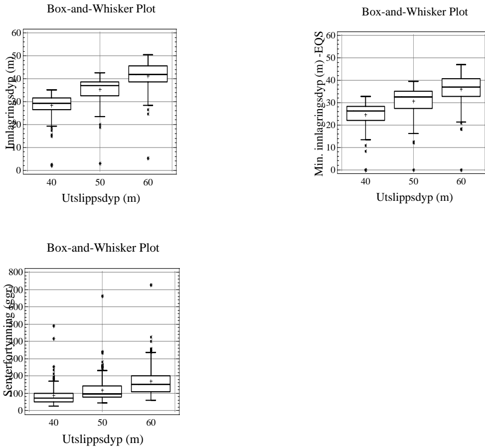
Figur 10. Innlagringsdyp og senterfortynning ved utslipp på 40, 50 og 60 meters dyp. Hulldiameter 0.1 m og hullhastighet = 1.5 m/s. Analysen er basert på samtlige observasjoner fra Bekkelagsbassenget i tidsrommet 1962-97.
