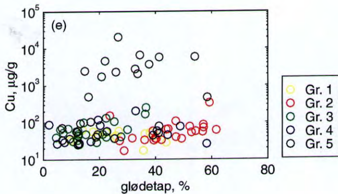
Figur 7. Kobber i innsjøsedimenter
