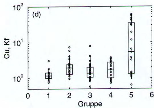
Figur 7. Kobber i innsjøsedimenter
