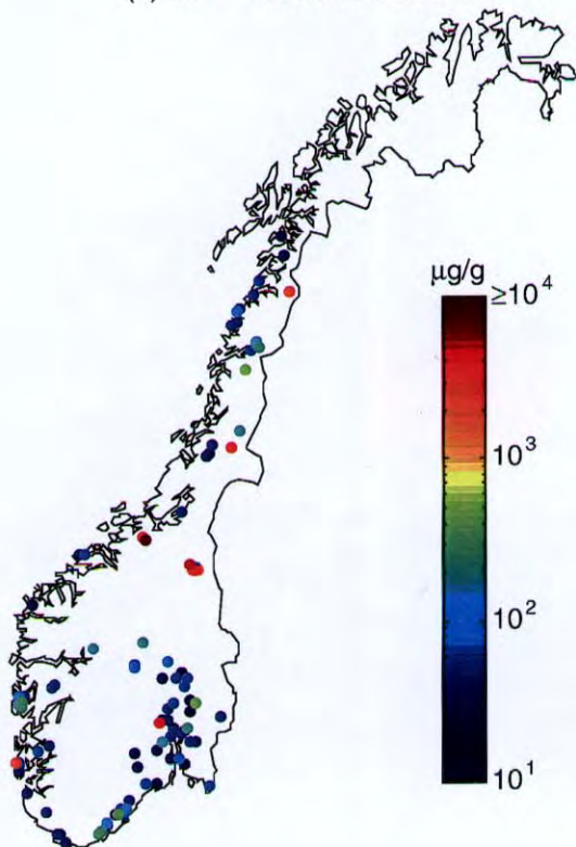
(a) Cu — overflatesedimenter
