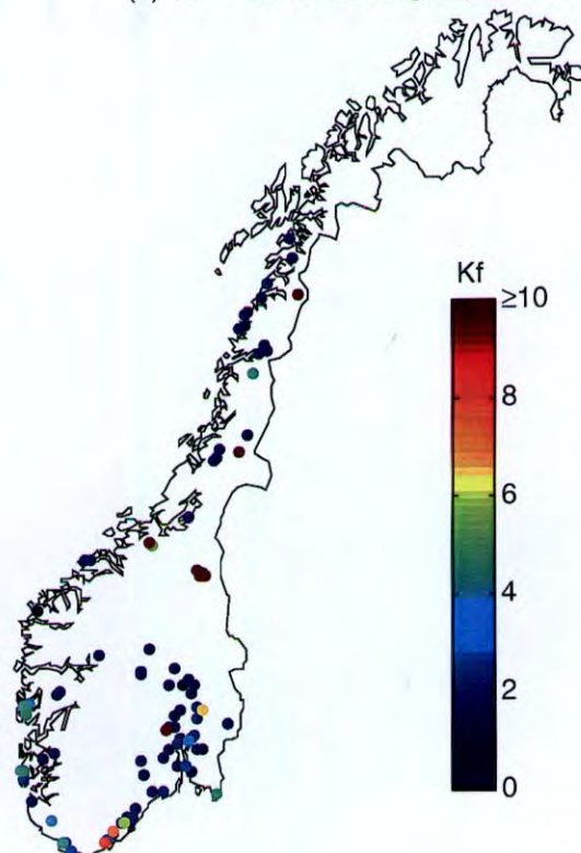
(b) Cu — kontamineringsfaktor
