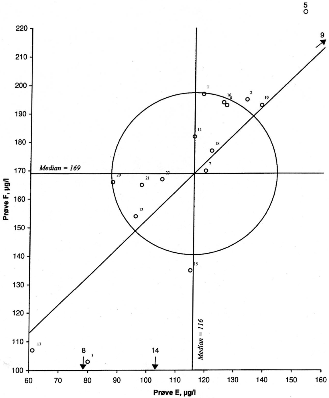
Figur 3. Youdendiagram for sølv, Prøvepar EF Akseptansegranse er 20 % , vist ved sirkelen
