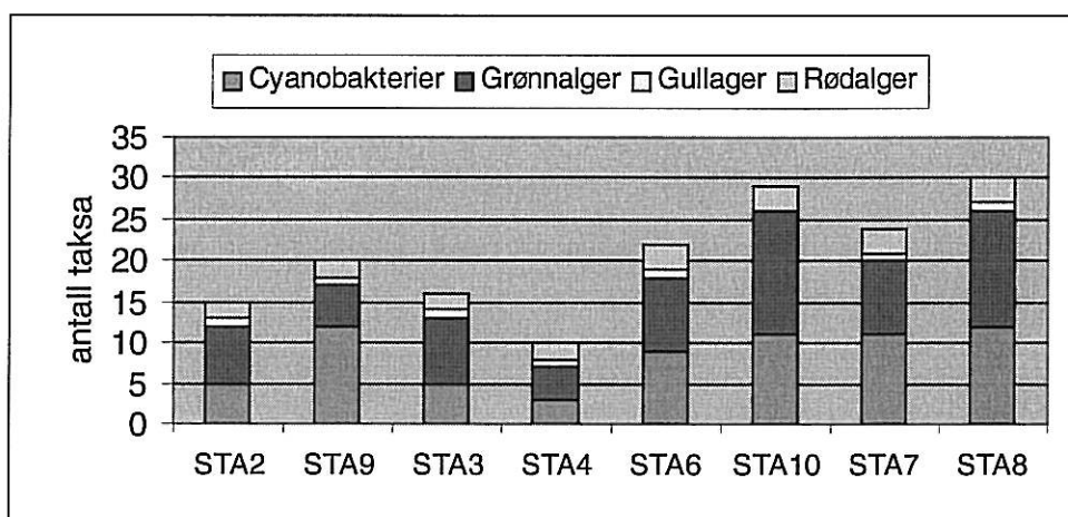
Figur 12. Totalt mangfold av alger (unntatt kiselalger) registrert på stasjoner i Surna og sideelvene Rinna (st.9) og Vindøla (st.10) i juni/juli og september 1998. Mangfold angitt som antall taksa (antall arter og grupper av arter).
