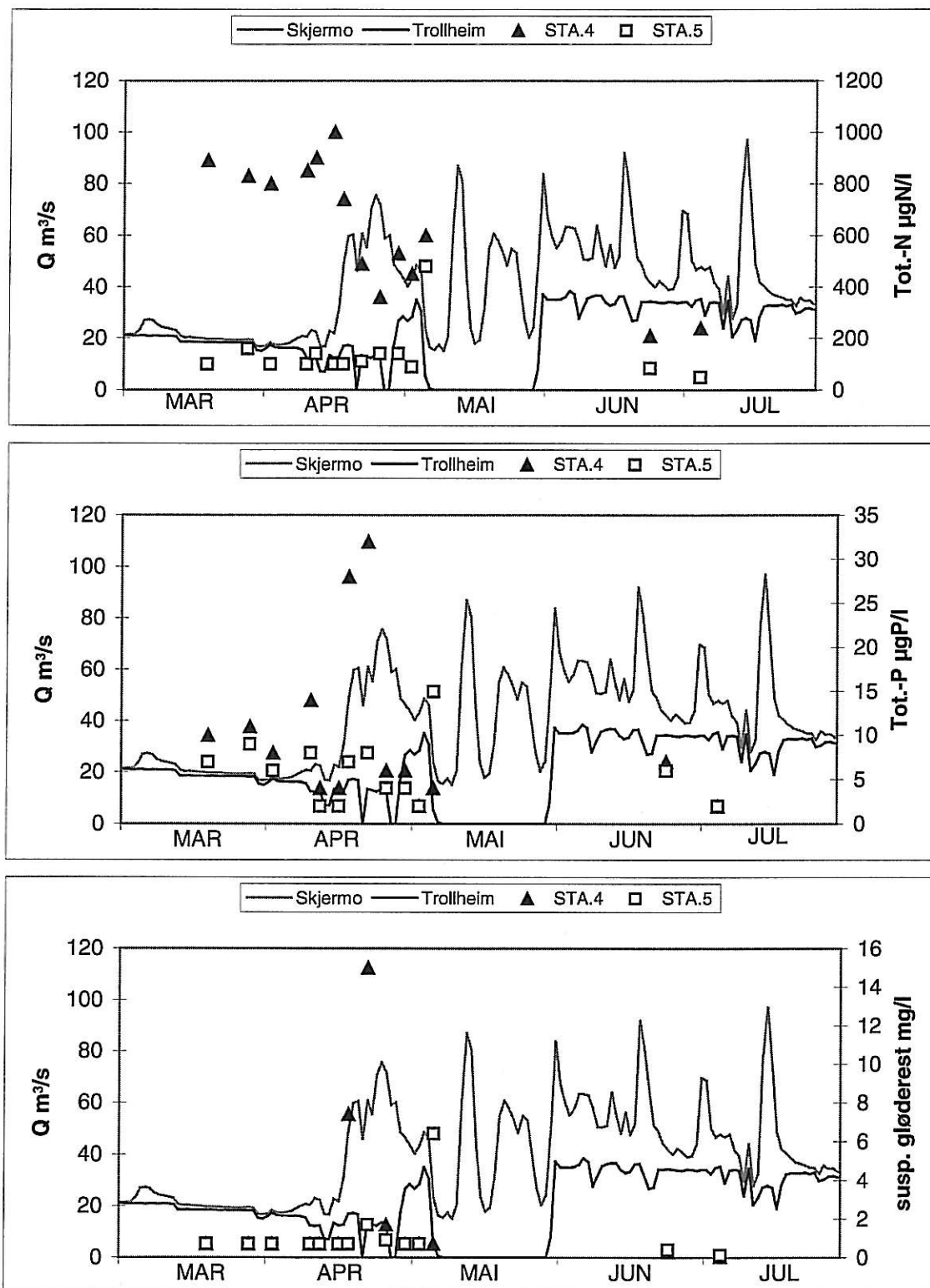
Figur 11. Målte verdier for total nitrogen (Tot.-N), total fosfor (Tot.-P) og suspendert gløderest i vannprøver fra to stasjoner i Surna i perioden mars-juli 1996 i forhold til vannføring ved Skjermo og driftsvannføring i Trollheim kraftverk. Sta 4 = Surna rett oppstrøms utløp Trollheim, sta.5 = utløpsvann fra Trollheim kraftverk.
