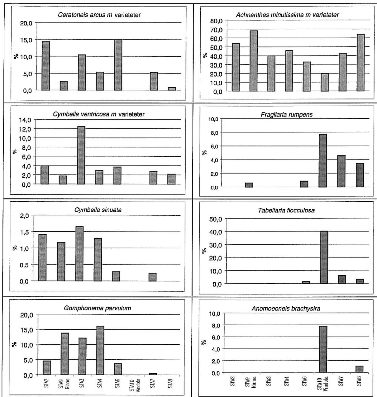
Figur 15. Prosentvis forekomst av noen kiselalger i Surna og sideelvene Rinna og Vindøla. 15. september 1998. NB ! Algene har ulik skala for prosentvis forekomst.
