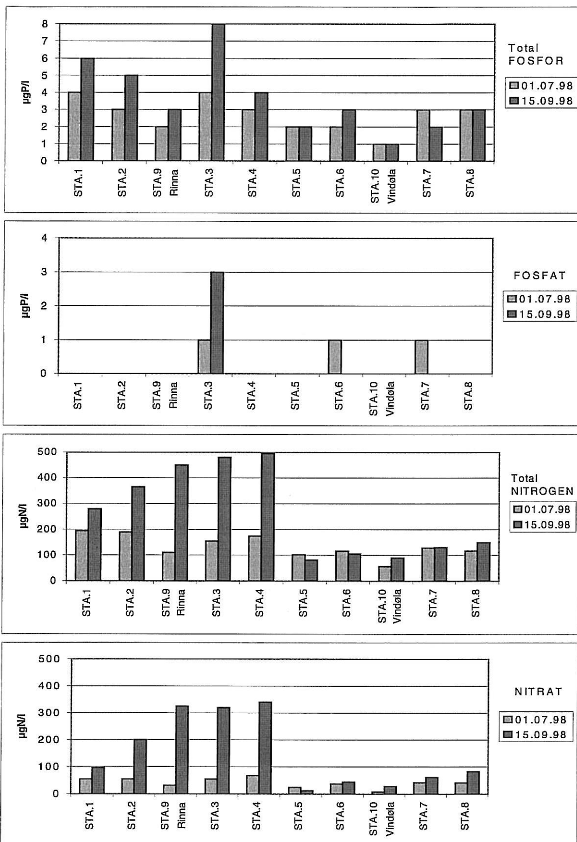
Figur 8. Enkeltmålinger av Tot.-P, fosfat, Tot.-N og nitrat på 10 stasjoner i Surnavassdraget 1.juli og 15.september 1998.
