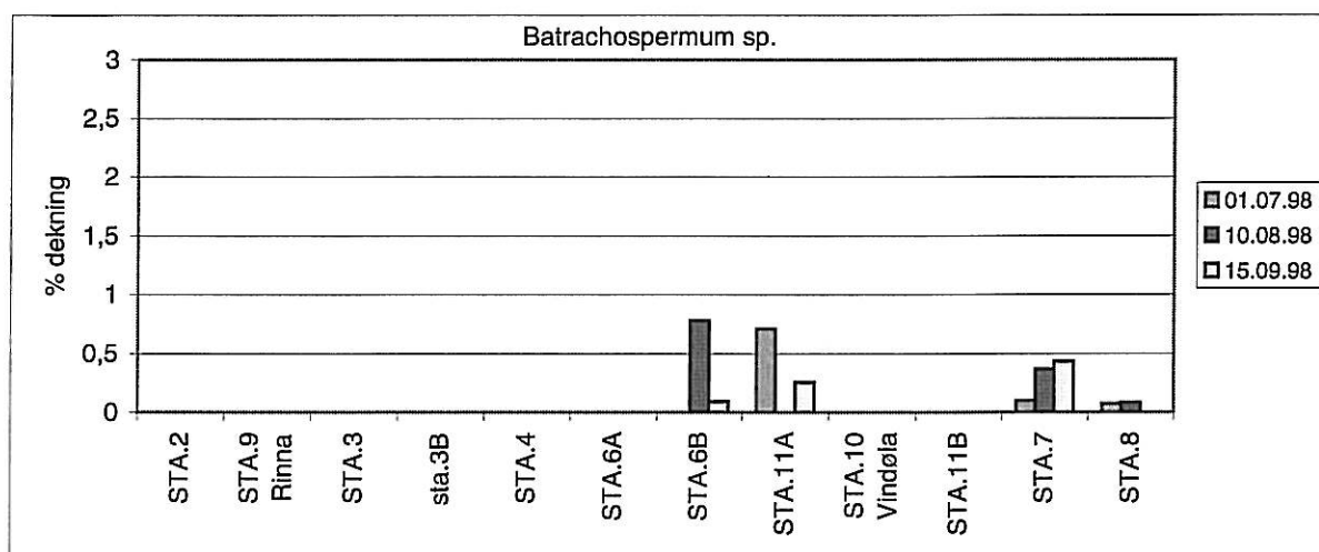
Figur 25. Prosent dekning av Batrachospermum sp. på 12 stasjoner i Surnavassdraget i 1998.
