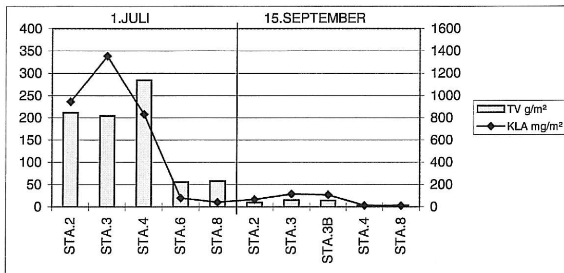
Figur 18. Biomasseprøver av trådformede grønnalger i Surna 1. juli og 15. september 1998. Biomasse mål som tørrvekt (TV g/m 2 ) og klorofylltetthet (KLA mg/m 2 ).
