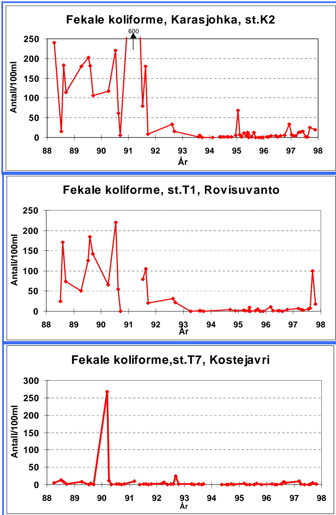
Figur 3.1. Fekale koliforme bakterier ved Karasjohka (K2), Rovisuvanto (T01) og Kostejavri (T07), 1988 -1997.
