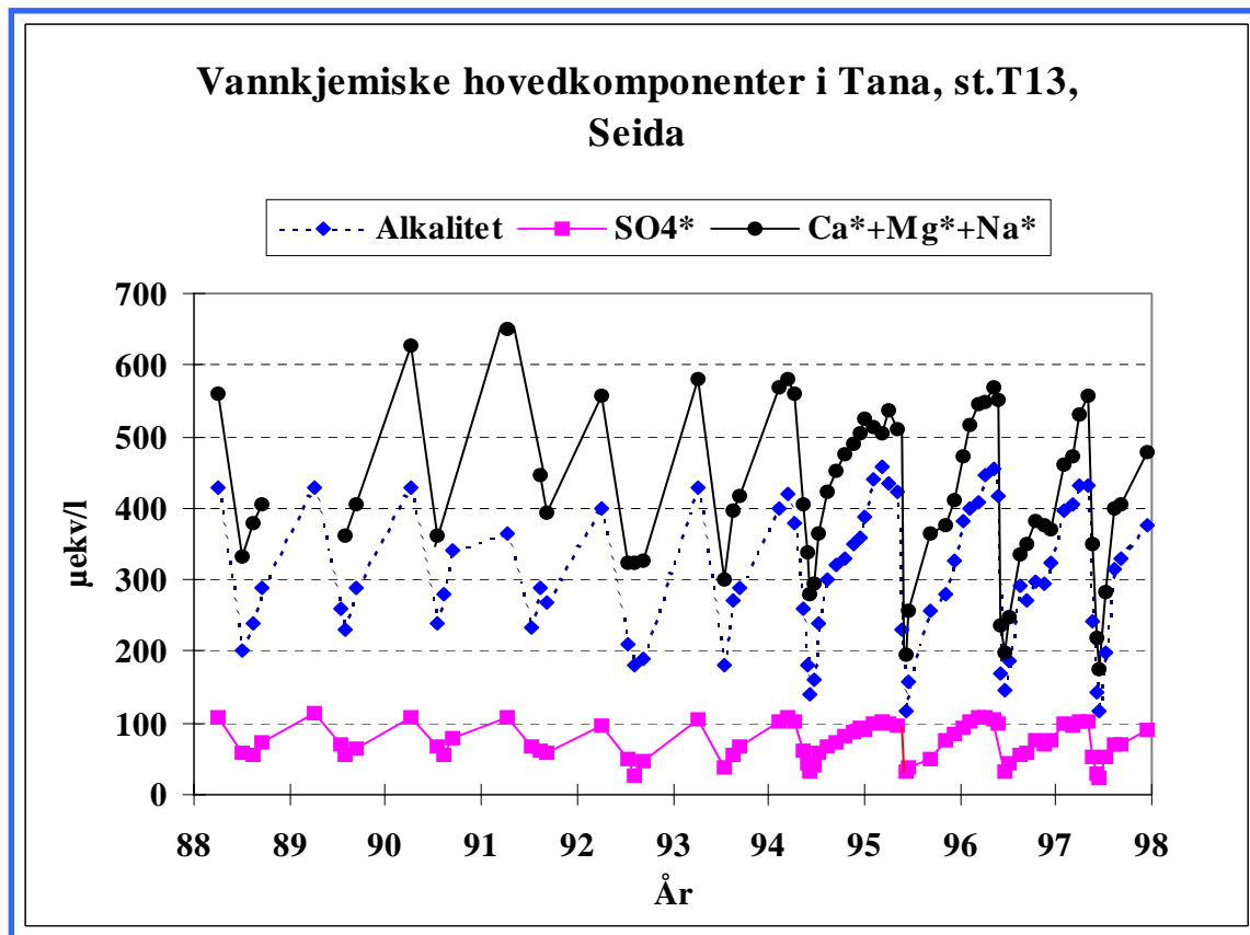
Figur 2.1. Vannkjemiske hovedkomponenter i Tana ved Seida (T13) for perioden 1988-1997. \text{Ca}^* + \text{Mg}^* + \text{Na}^* (sjøsaltkorrigert), \text{SO}_4^* (sulfat, sjøsaltkorrigert) og alkalitet.
