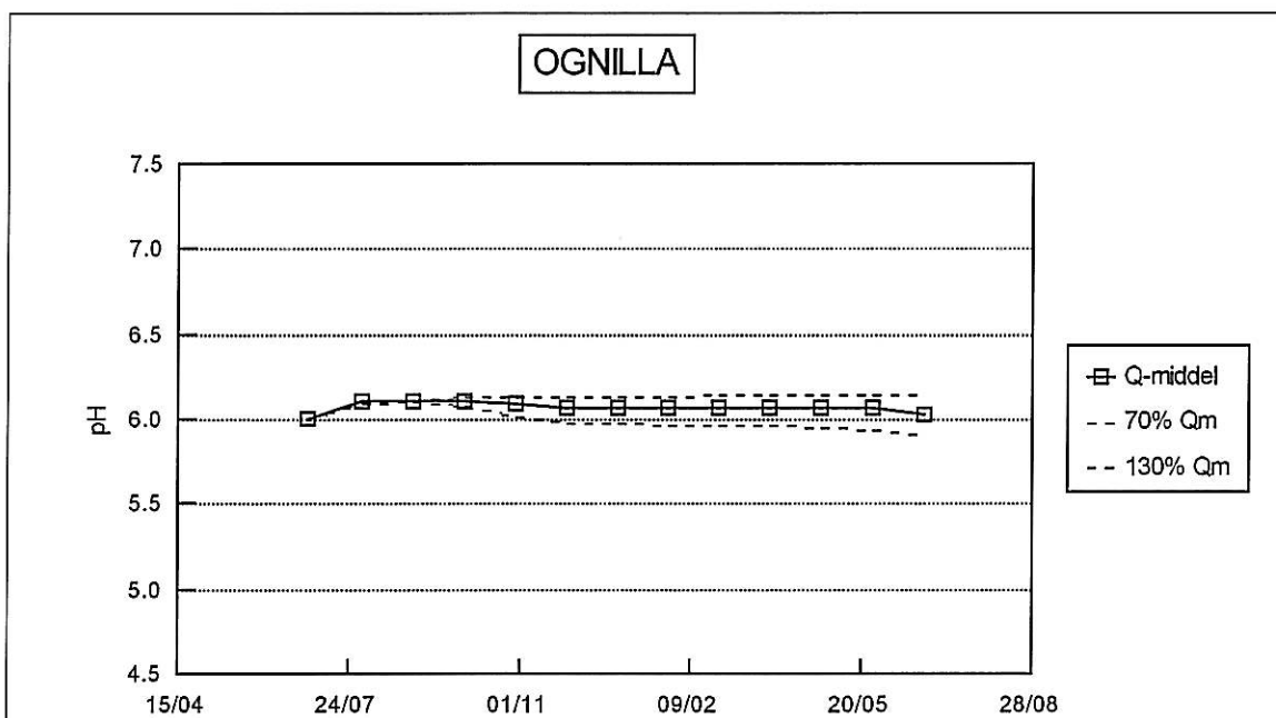
Figur 4. Vannkvalitetsutviklingen i Ognilla ved simulert omkalking (hel linje med firkanter; annen gangs kalking med totalt 38 tonn). 70 % av normal avrenning gir et forløp med høyere pH, mens 130 % gir lavere pH enn ved normal avrenning (Q-middel).
