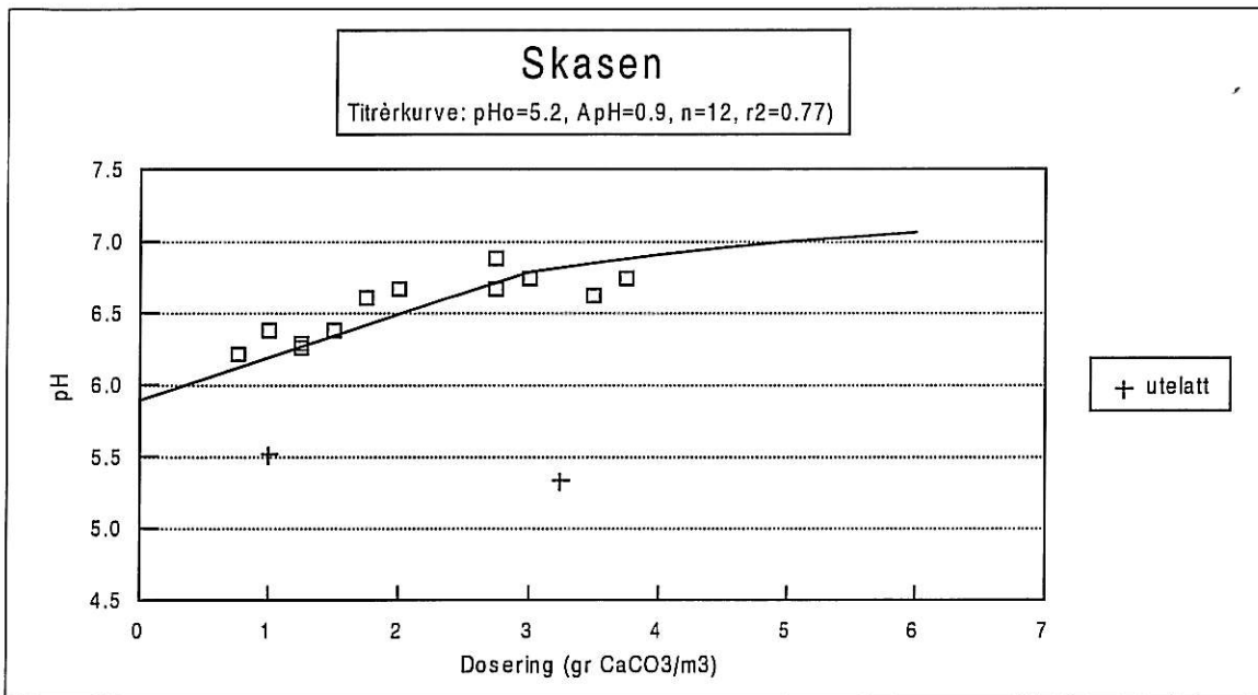
Figur 1. Sammenhengen mellom pH og oppløst CaCO 3 . Beregningen av tilsatt mengde CaCO 3 er gjort på grunnlag av Ca-data for innsjøen. Forklaring av kurvekarakteristika (pH o og A pH ) er gitt i Håøya et al. (1996). Målinger som sannsynligvis er feil analysert eller ikke representative for vannkvalitetsutviklingen er vist med symbolet +.
