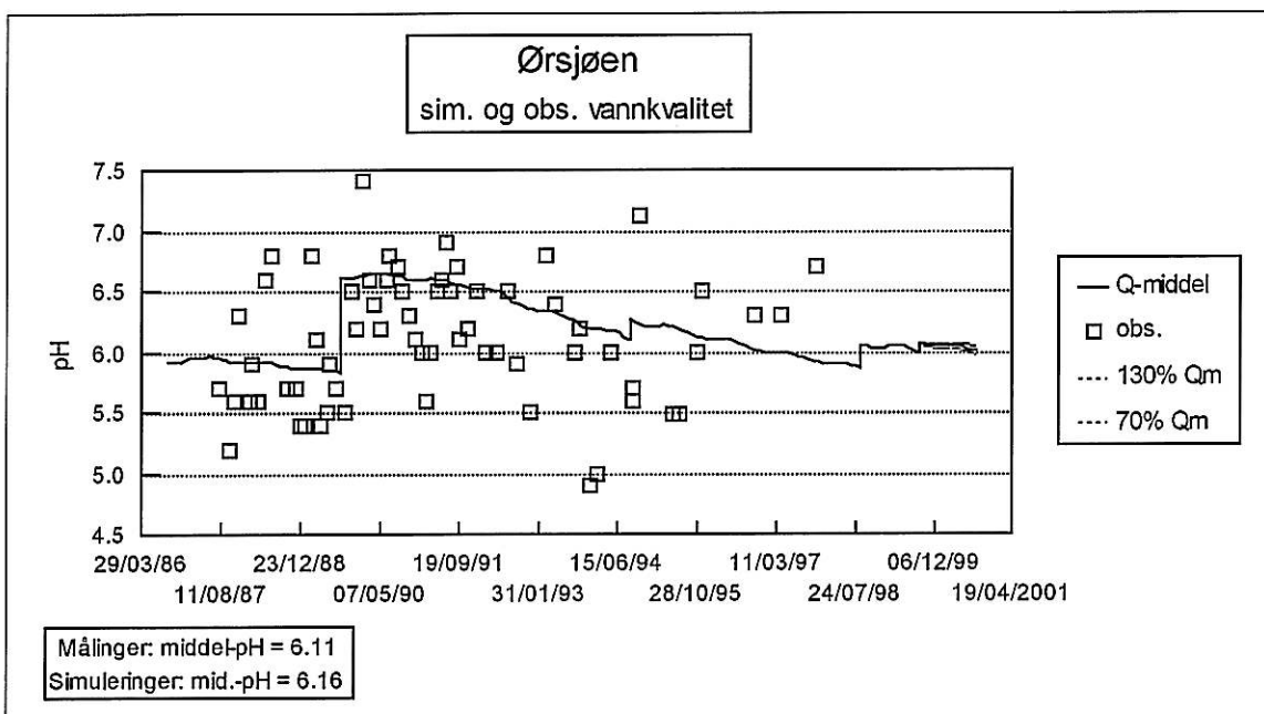
Figur 9. Målt pH (firkanter) og simulert pH-utvikling (hel linje) på basis av midlere avrenning (Q-middel) i Ørsjøen. Bemerk den store spredningen i pH-målingene, se teksten. Den innlagte variasjonen i avrenning hadde ingen betydning for simuleringsforløpet.
