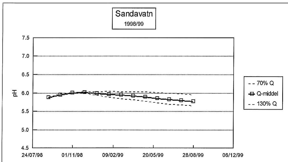
Figur 33. Simuleringer av forutsatt kalking av Sandavatn i 1998. 130 % av normal avrenning gir noe lavere pH ved omkalking.
