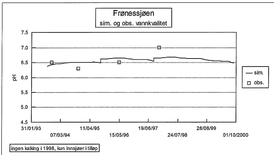
Figur 7. Målt pH (firkanter) og simulert pH-utvikling (hel linje) på basis av midlere avrenning (Q-middel) i Frønessjøen 1993-2001. Det er kun forutsatt kalking av innsjøene oppstrøms f.o.m. 1998.
