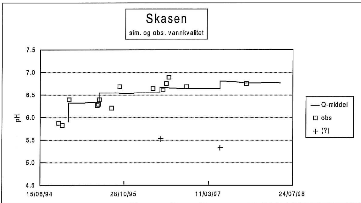
Figur 2. Målt pH (firkanter) og simulert pH-utvikling (hel linje) på basis av midlere avrenning (Q-middel) i Skasen. Målinger som kan være feil analysert eller ikke representative for vannkvalitetsutviklingen er vist med symbolet +.
