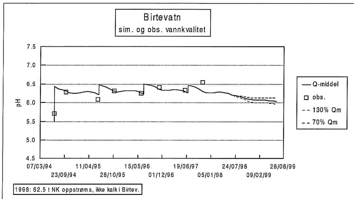
Figur 17. Målt pH (firkanter) og simulert pH-utvikling (hel linje) på basis av midlere avrenning (Q-middel), både for utført og planlagt (1998) kalking i Birtevatn. Vatnet trenger ikke kalk i 1998, forutsatt kalking av de fleste innsjøene i tilløp med tilsammen 62.5 t NK-kalk.
