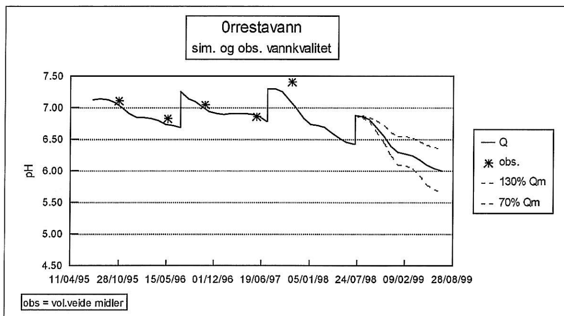
Figur 26. Målt pH (stjerner) og simulert pH-utvikling (hel linje) på basis av midlere avrenning (Q-middel) i Orrestadvatn. 130 % av normal avrenning kan gi pH ned mot 5.7 før omkalking. Merk at målingene er volumveide middelverdier for innsjøen.
