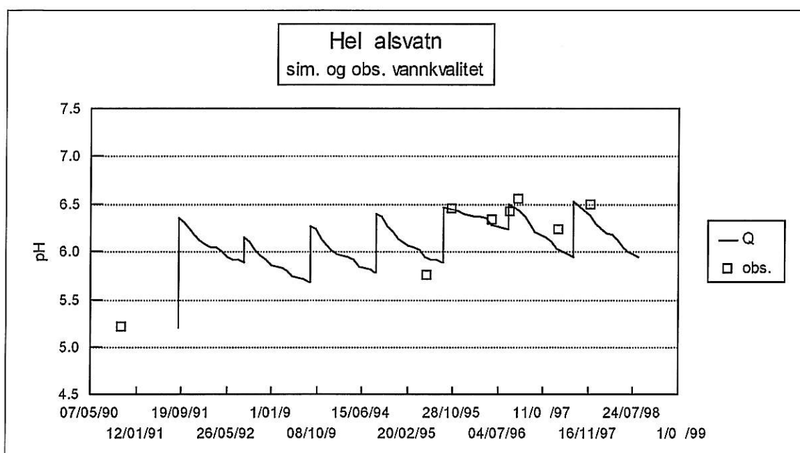
Figur 29. Målt pH (firkanter) og simulert pH-utvikling (hel linje) på basis av midlere avrenning (Q-middel) i Heldalsvatn fram til 1998 (1998-kalkingen er vist i Figur 30 ).
