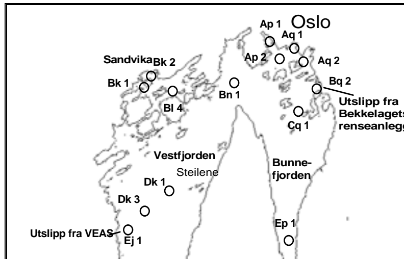
Figur 3. Overflatestasjoner juni-august 1998.
