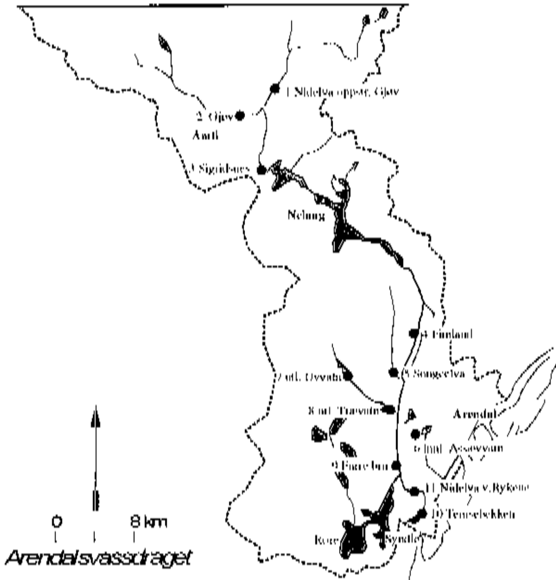
Figur 9. Nedre del av Arendalsvassdraget med prøvetakingsstasjoner som fungerer i rullerende overvåking i Aust-Agder vassdrag (fra Kuste og Håvardstam 1999).
