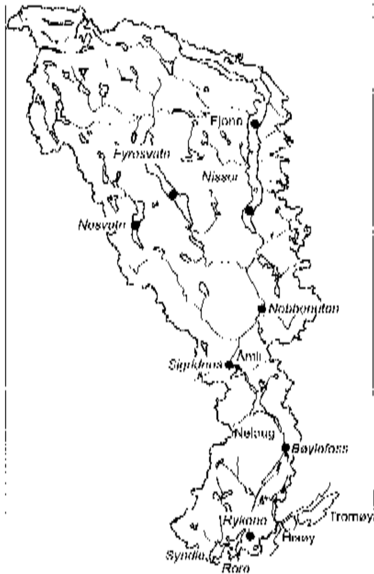
Figur 3. Nedbørfeltet til Arendalvassdraget med prøvetakingssjøsjoner for vannkjemisk inntegrert.
