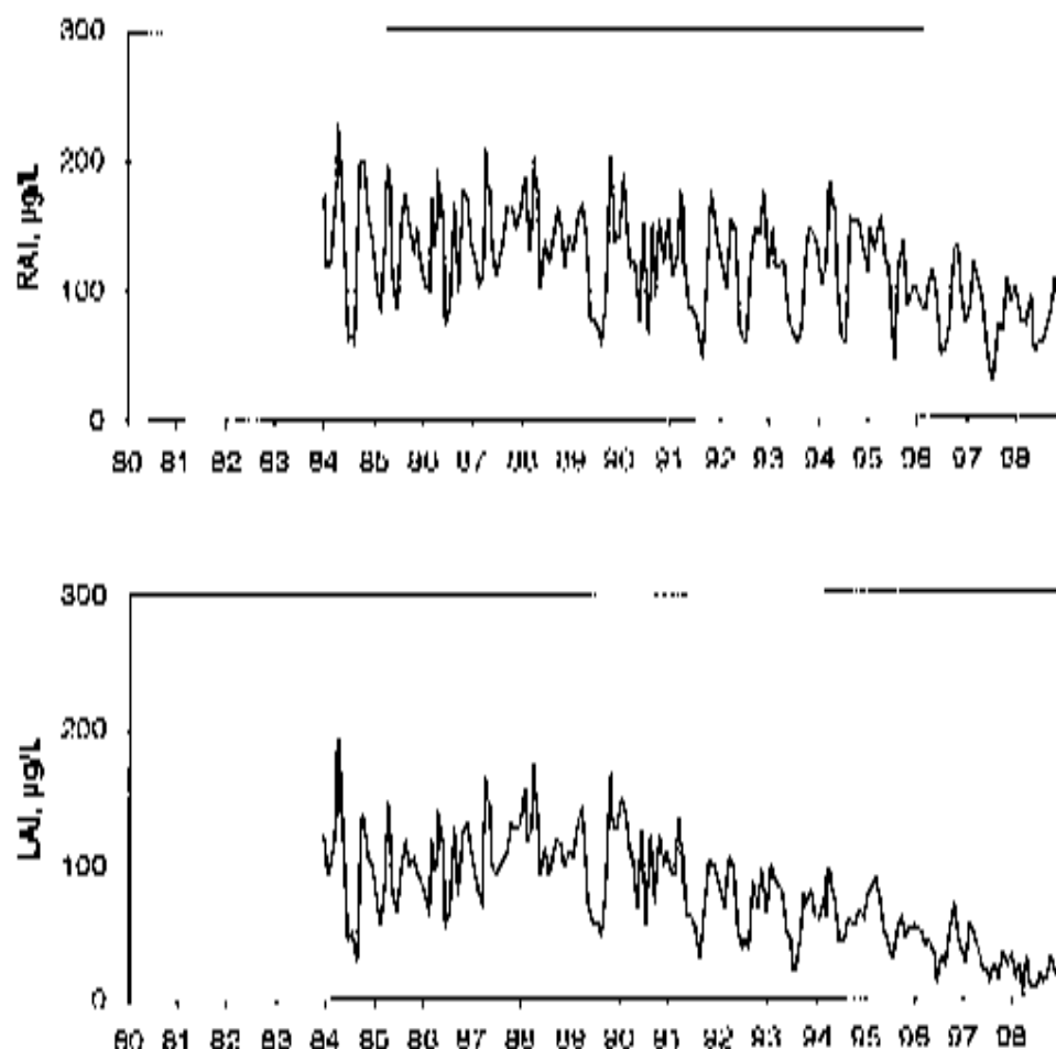
Figur 7. Utviklingen i reaktivt og labilt aluminium i perioden 1980-1998. Data fra DN og NITs overvåkingsprogram.
