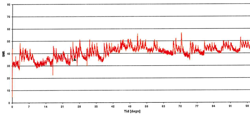
Figur 11. SNR-verdier på a) 3, b) 6, c) 9 og d) 12 meters dyp i måleperioden på Stasjon A utenfor dumpingsområdet.
