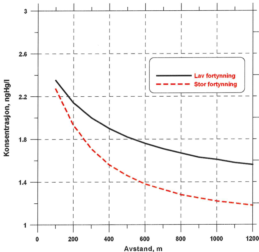
Figur 12. Beregnet konsentrasjon av kvikksølv i sentrum av en sky med oppvirvlet bunnsedimenter, med økende avstand fra kanten av siltskjørtet. En kurve viser beregningene ved antatt lav fortykning (konstant turbulent diffusjonskoeffisient) og en annen viser resultater for antatt stor fortykning (turbulent diffusjonskoeffisient som øker med tiden). Nygårdsbroen ligger ca. 700 m fra kanten av siltskjørtet, som det lå den 30.3.99.
