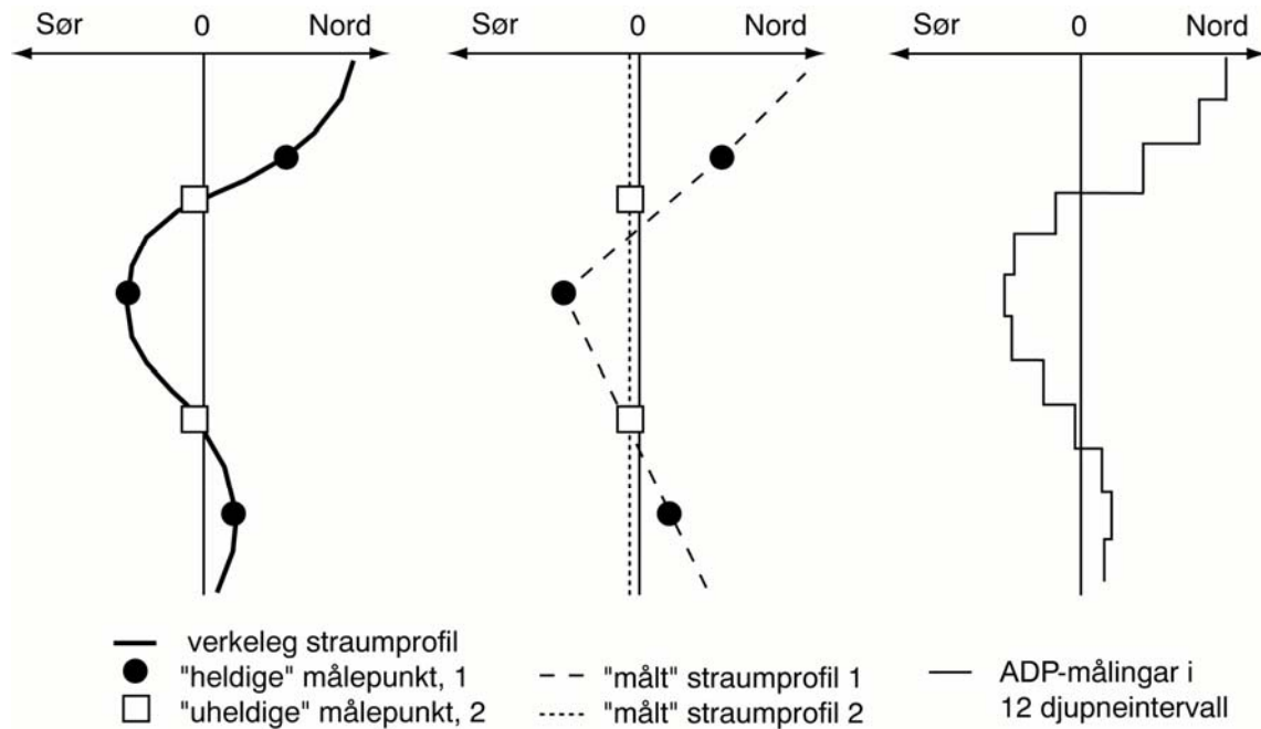
Figur 4. Prinsippskisse som syner "sant" strømsprofil og "målte" profiler basert på ulike antal målepunkt i vertikalen, og ulik plassering av desse. Dersom måledjupa (eller målecellene for ein ADP) fell saman med sjikt der strømmen er sterkast, vil ein kunne få eit godt bilete av tilhøva, mens måling berre i sjikt med svak strøm vil gi eit feil bilete. Med fleire målepunkt eller djupneceller tilnærmar målt profil seg til "sant" profil.
