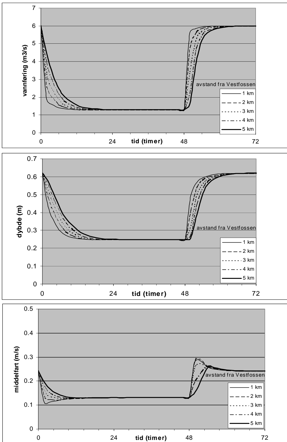
Figur 3.5 Respons i Vestfosselva ved 6 m 3 /s avbrutt av langvarig minstevannføring
