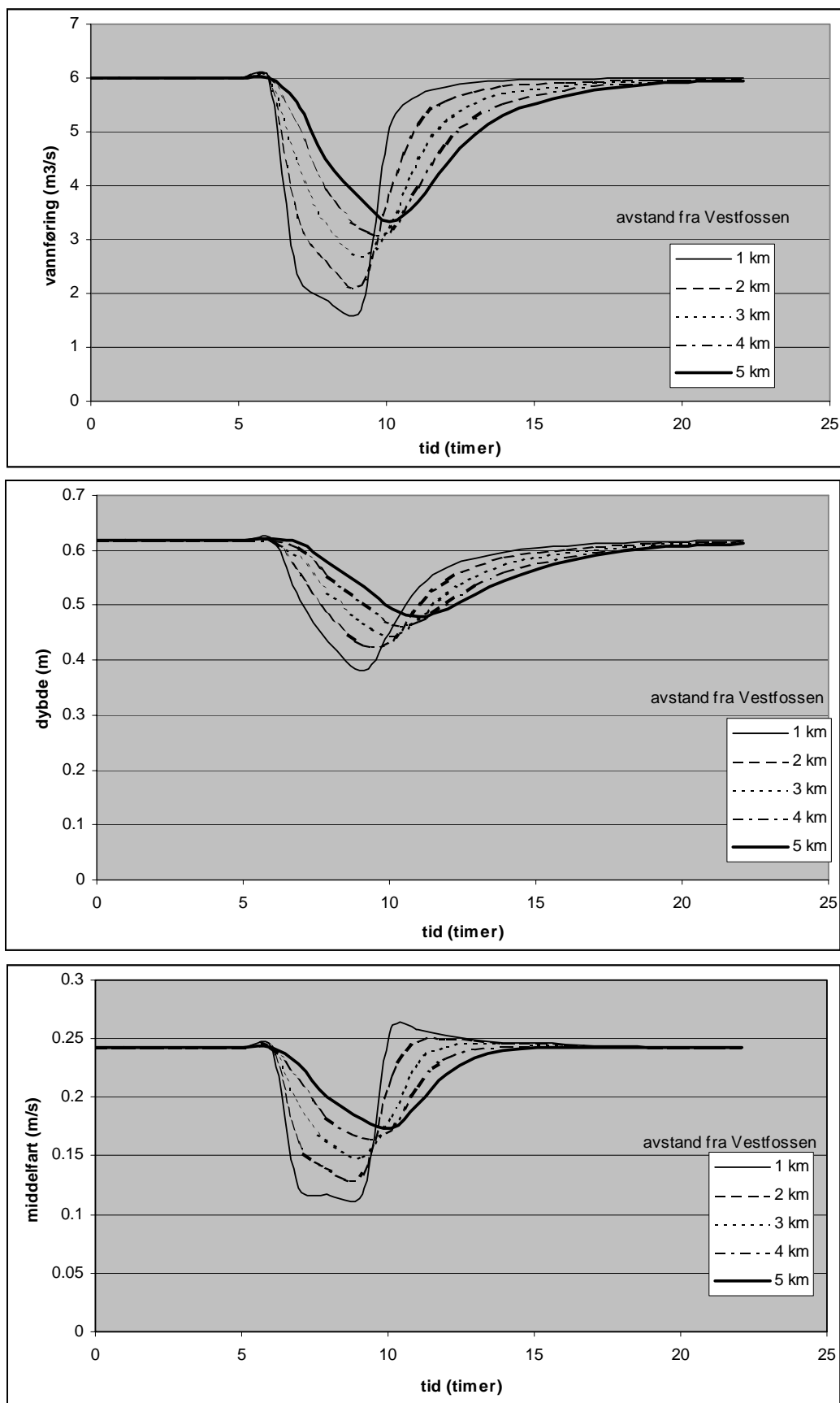
Figur 3.6 Respons i Vestfosselva ved 6 \text{ m}^3/\text{s} avbrutt av minstevannføring i 3 timer
