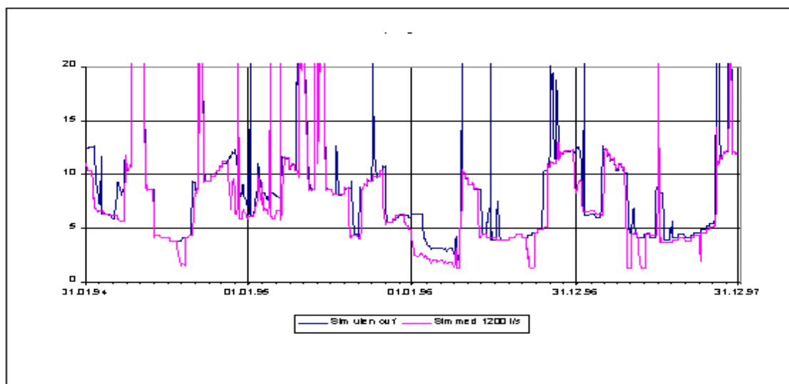
Figur 3.1 Simulert vannføring i Vestfosselva
