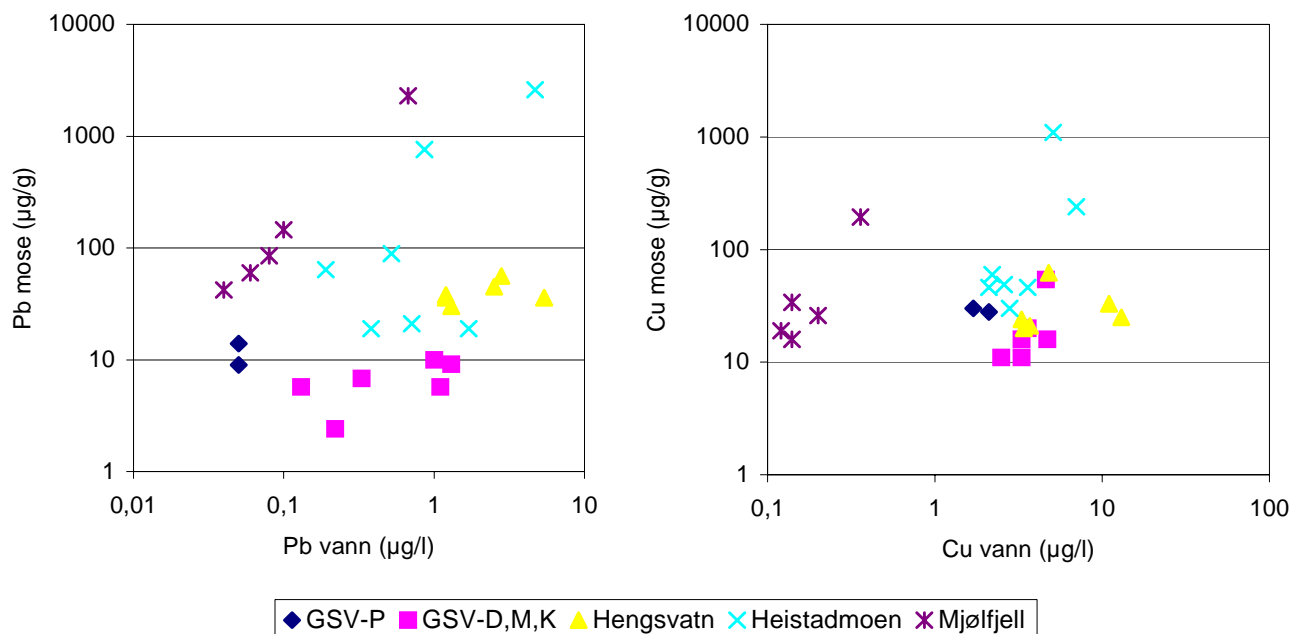
Fig. 15. Sammenhengen mellom konsentrasjonene av bly og kobber i vann og mose. Stasjonskoder på Høybuktkmoen (GSV) er gitt i Fig. 14.
