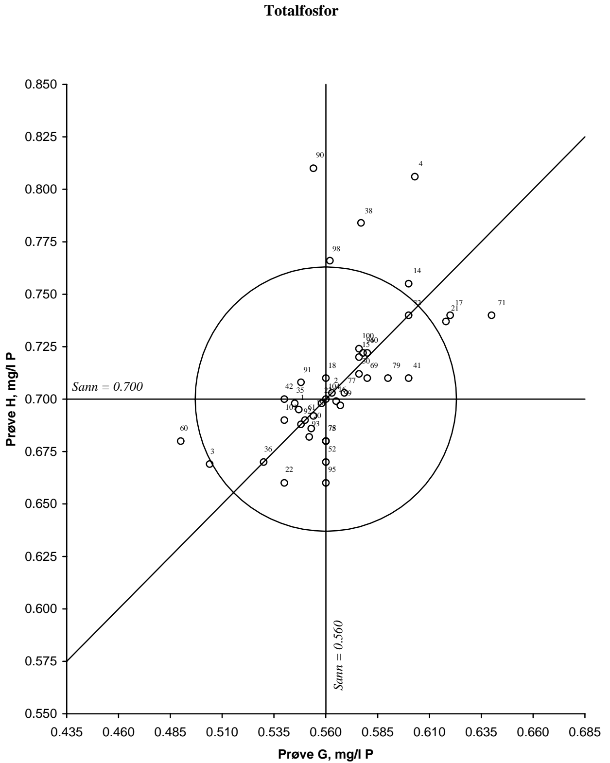
Figur 12. Youtenddiagram for totalfosfor, prøvepar GH Akseptansgrensen, angitt med en sirkel, er 10 %
