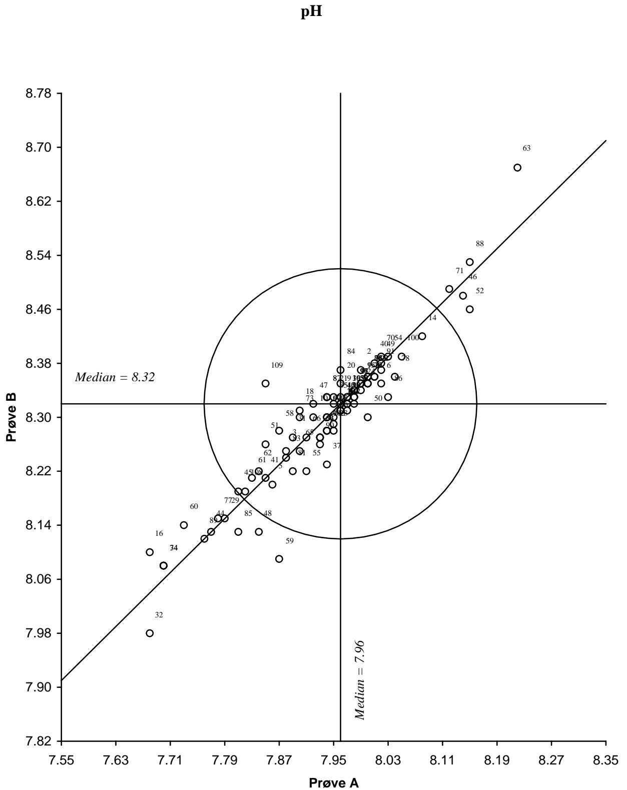
Figur 1. Youdendiagram for pH, prøvepar AB Akseptansesgrensen, angitt med en sirkel, er 0.2 pH enheter
