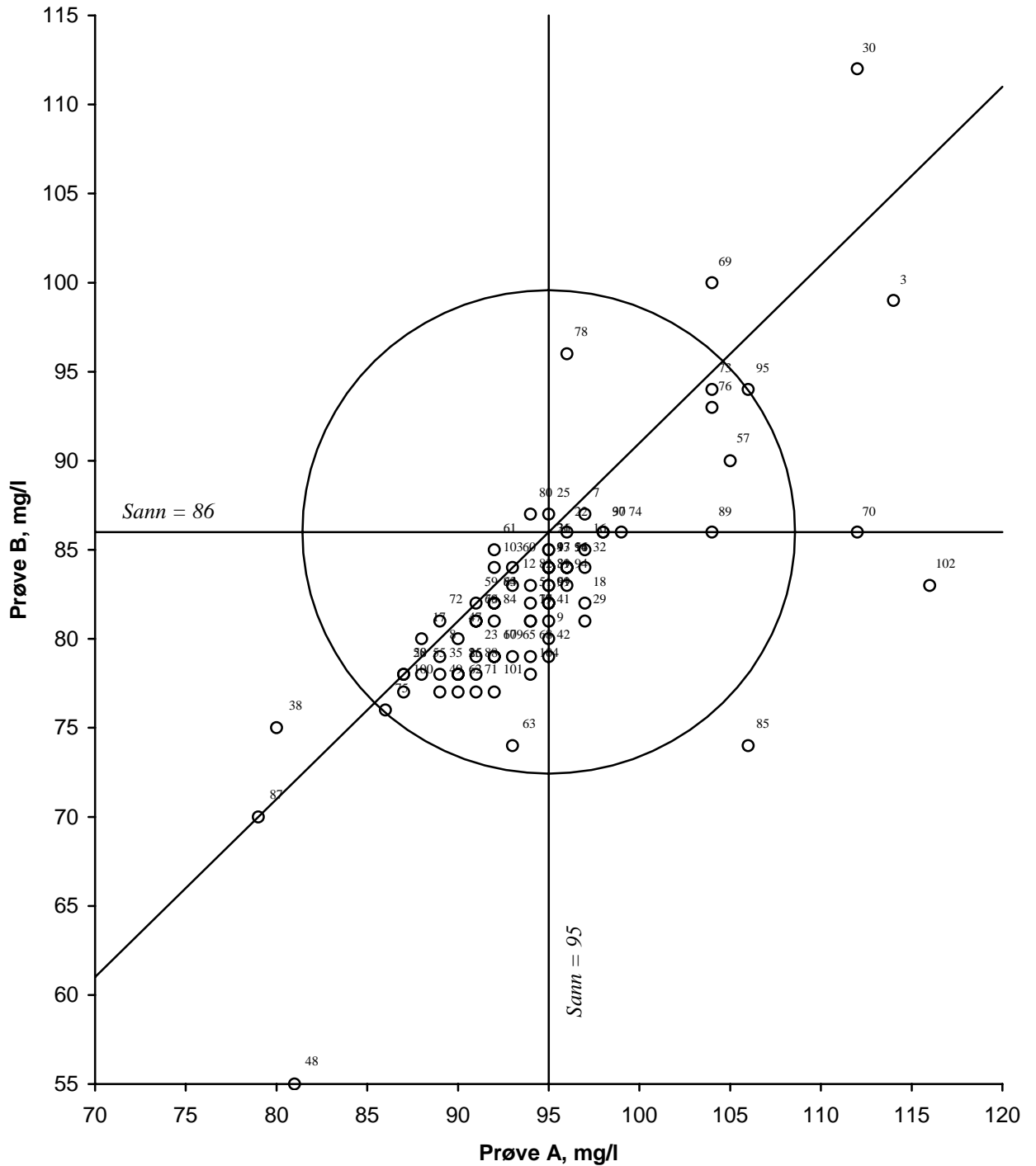
Figur 3. Youndendiagram for suspendert stoff, tørrstoff, prøvepar AB Akseptansegrensen, angitt med en sirkel, er 15 %
