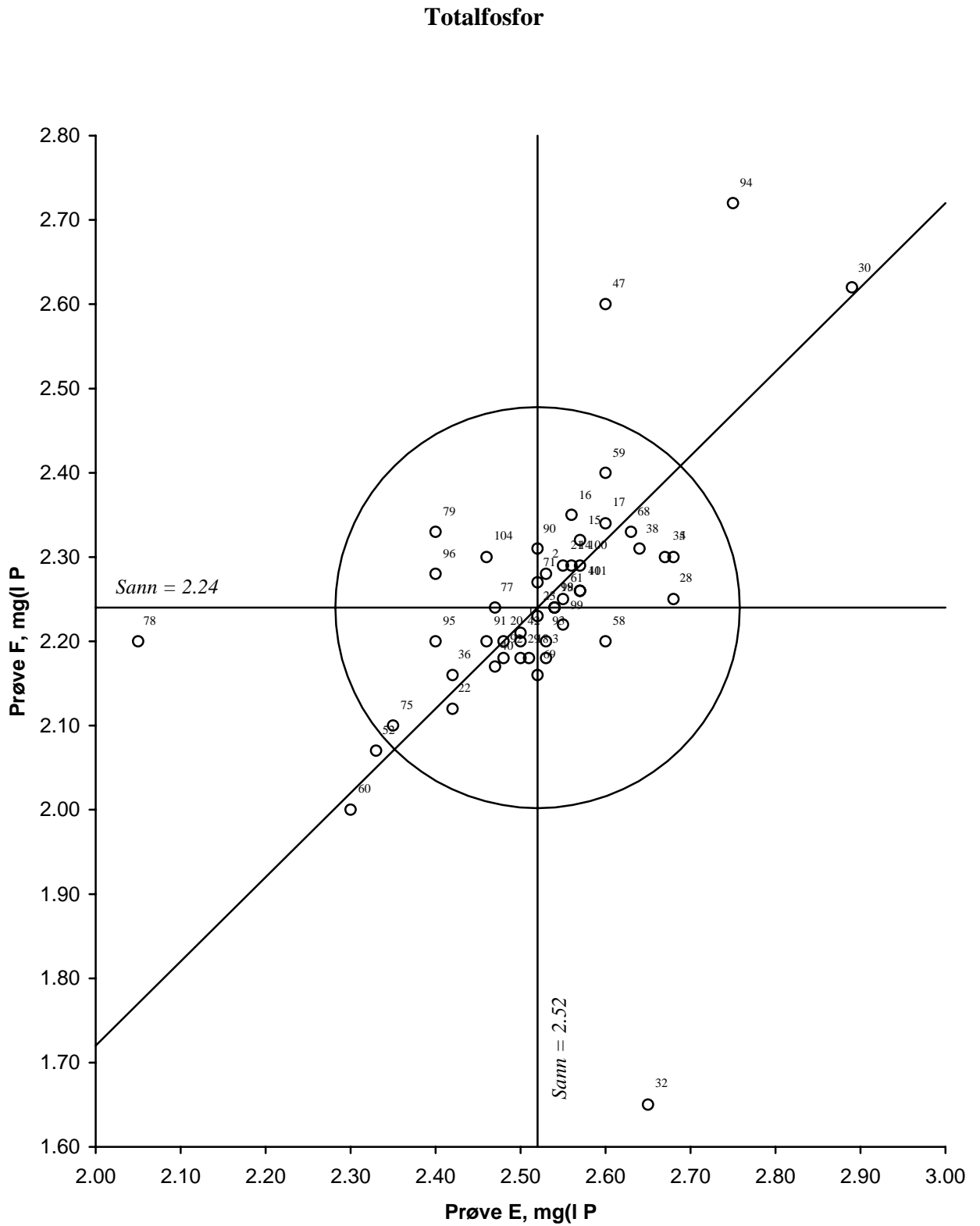
Figur 11. Youndendiagram for totalfosfor, prøvepar EF Akseptansegrensen, angitt med en sirkel, er 10 %
