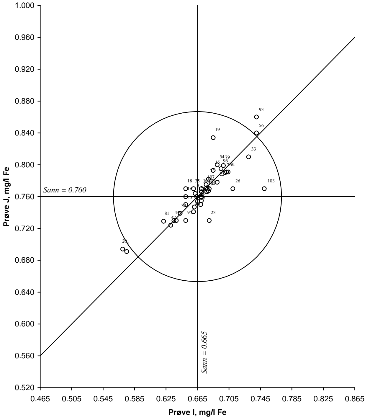
Figur 19. Youtendigram for jern, prøvepar IJ Akseptansgrensen, angitt med en sirkel, er 15 %
