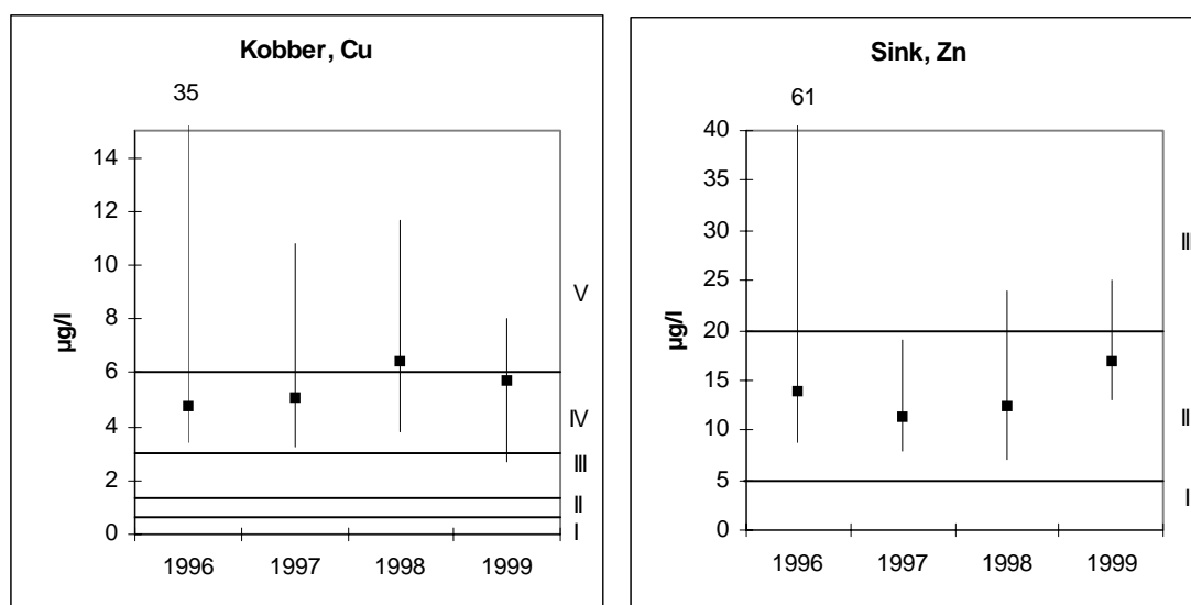
Figur 12. Konsentrasjoner av kobber og sink i Glåma ved Høyegga i 1996-99. Medianverdier og variasjonsbredder er vist. Tilstandsklasser er også markert i henhold til SFT's klassifikasjonssystem (SFT 1997). Klasse I-V tilsvarer henholdsvis "lite", "moderat", "markert", "sterkt" og "meget sterkt forurenset".
