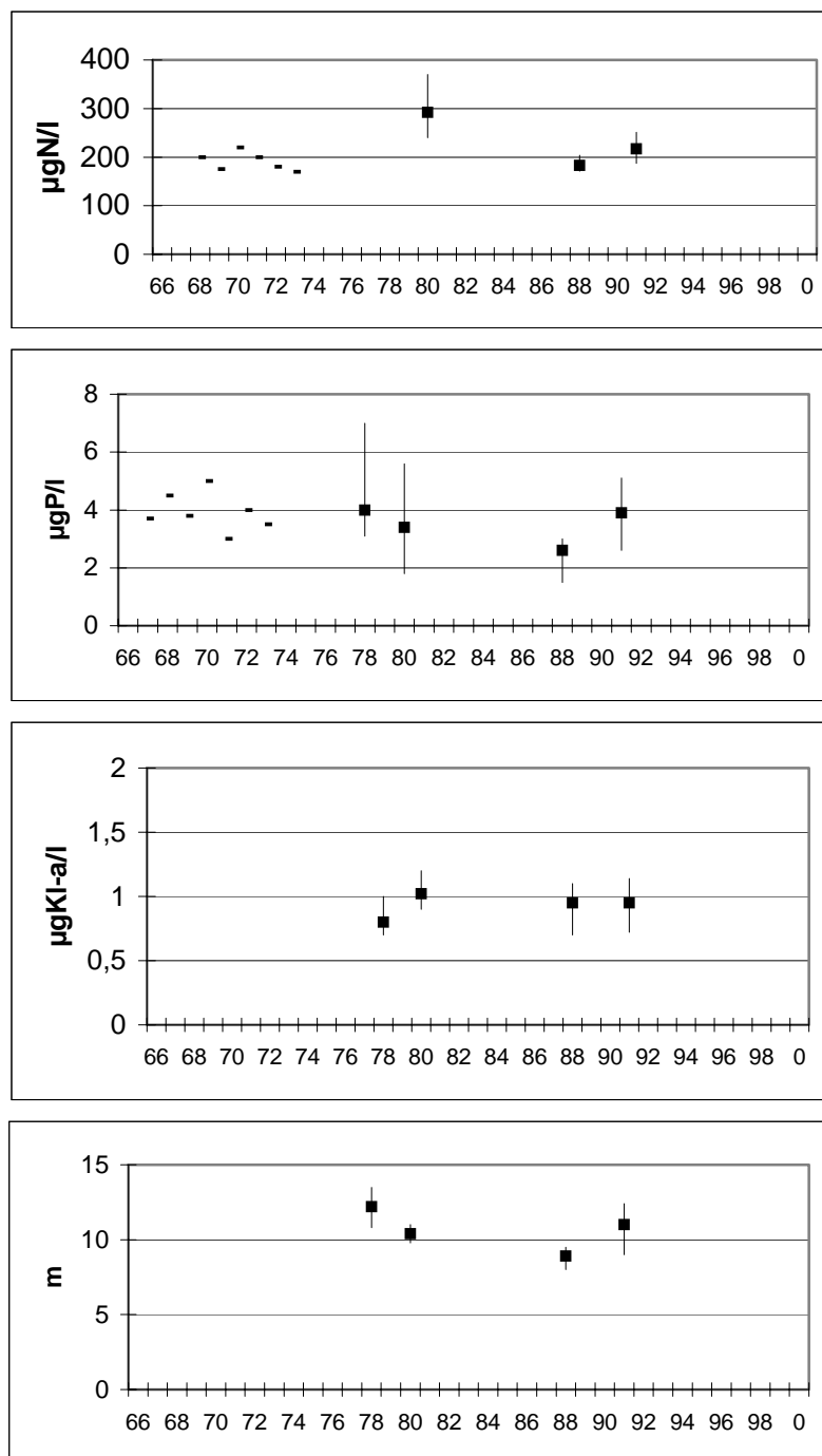
Fig. I. Femunden. Tidsutviklingen i konsentrasjoner av total-nitrogen, total-fosfor og klorofyll-a samt siktedyp. Middelerverdier og variasjonsbredder i vekstsesongen (juni-oktober) er vist bortsett fra for perioden 1967-73 hvor data fra vårsirkulasjonen er vist.
