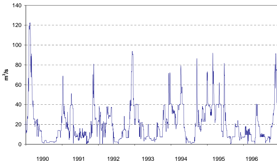
Figur 3. Vannføring i Tista (Tistefossen) 1990-1996.
