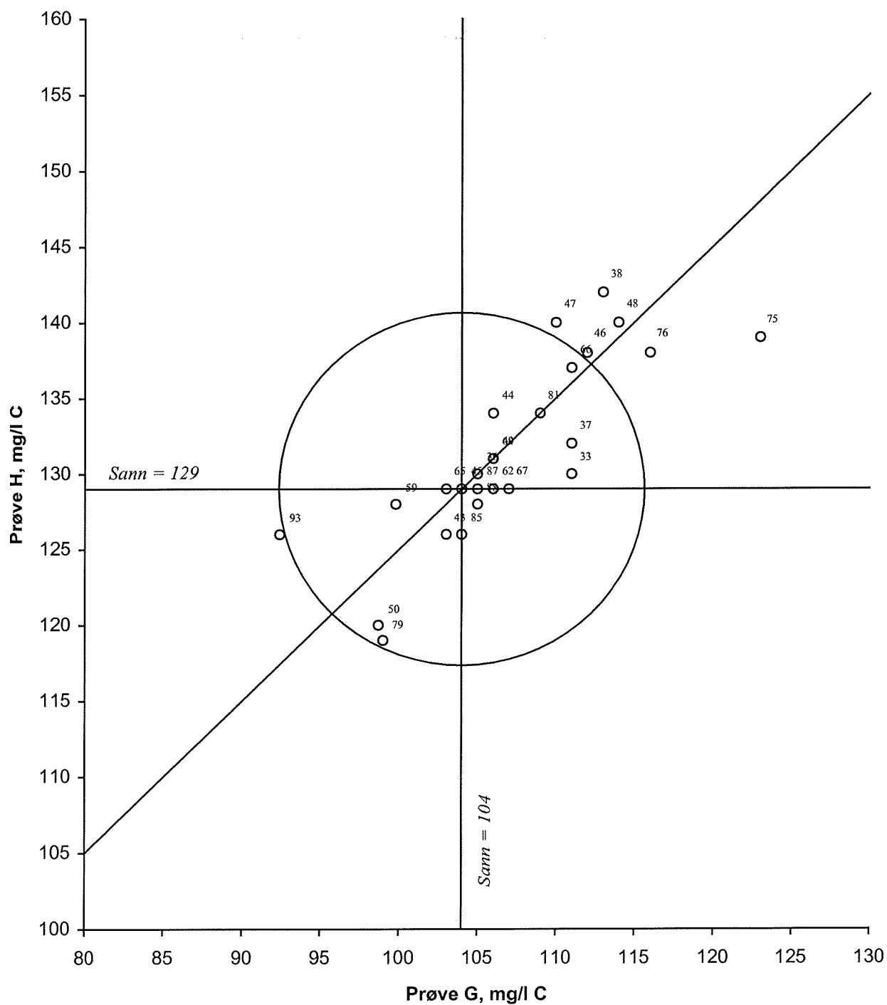
Figur 12. Youtenddiagram for totalt organisk karbon, prøvepar GH Akseptansegrensen, angitt med en sirkel, er 10 %
