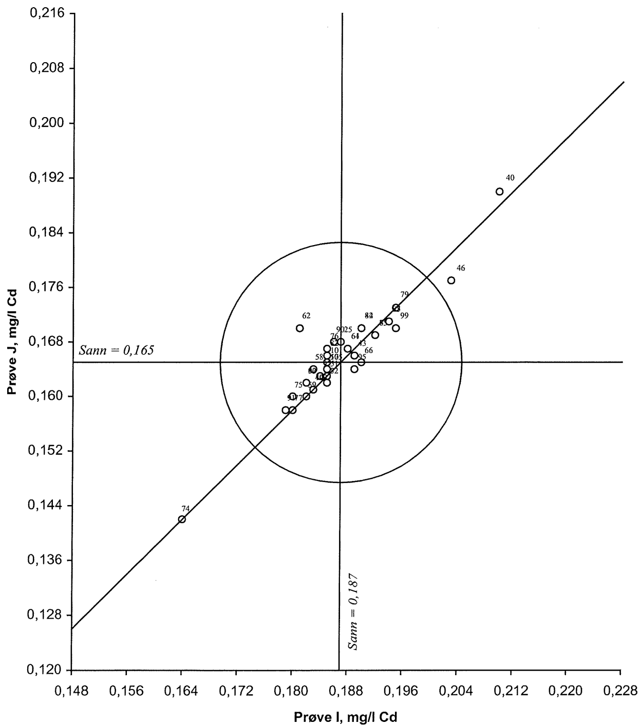
Figur 21. Youndendiagram for kadmium, prøvepar IJ Akseptansegrensen, angitt med en sirkel, er 10 %
