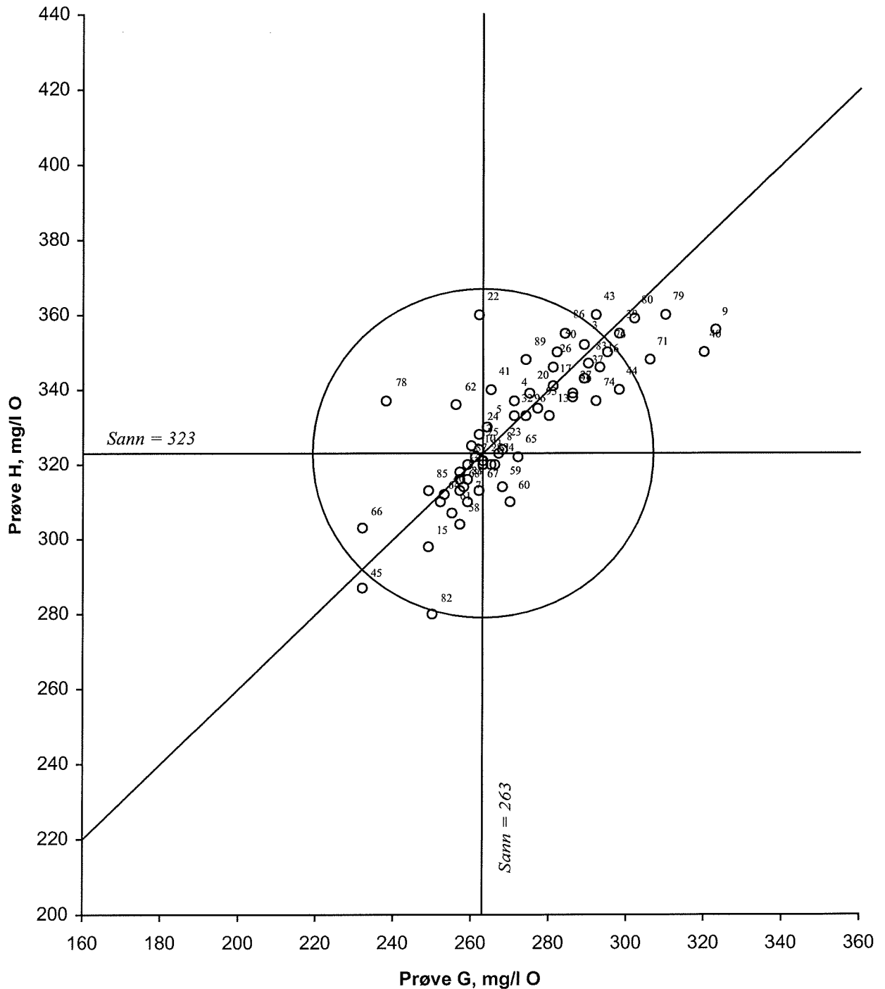
Figur 8. Youdendigram for kjemisk oksygenforbruk, COD/Cr, prøvepar GH Akseptansesegrensen, angitt med en sirkel, er 15 %
