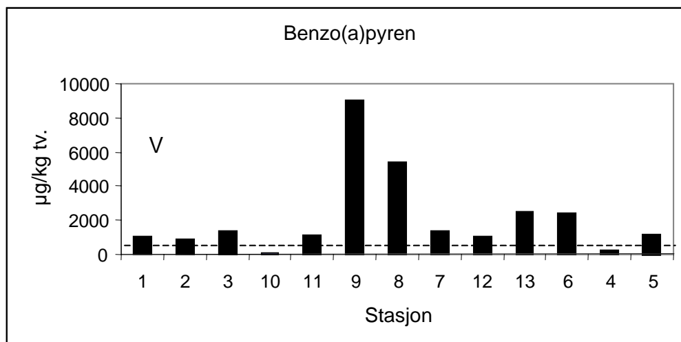
Figur 8. Konsentrasjoner av benzo(a)pyren i øvre 0-2 cm av sedimentet. Stasjonene er sortert fra SV til NØ langs land. Grenseverdi mellom klasse IV og V i SFTs miljøkvalitets-klassifisering er angitt med stiplet linje.
