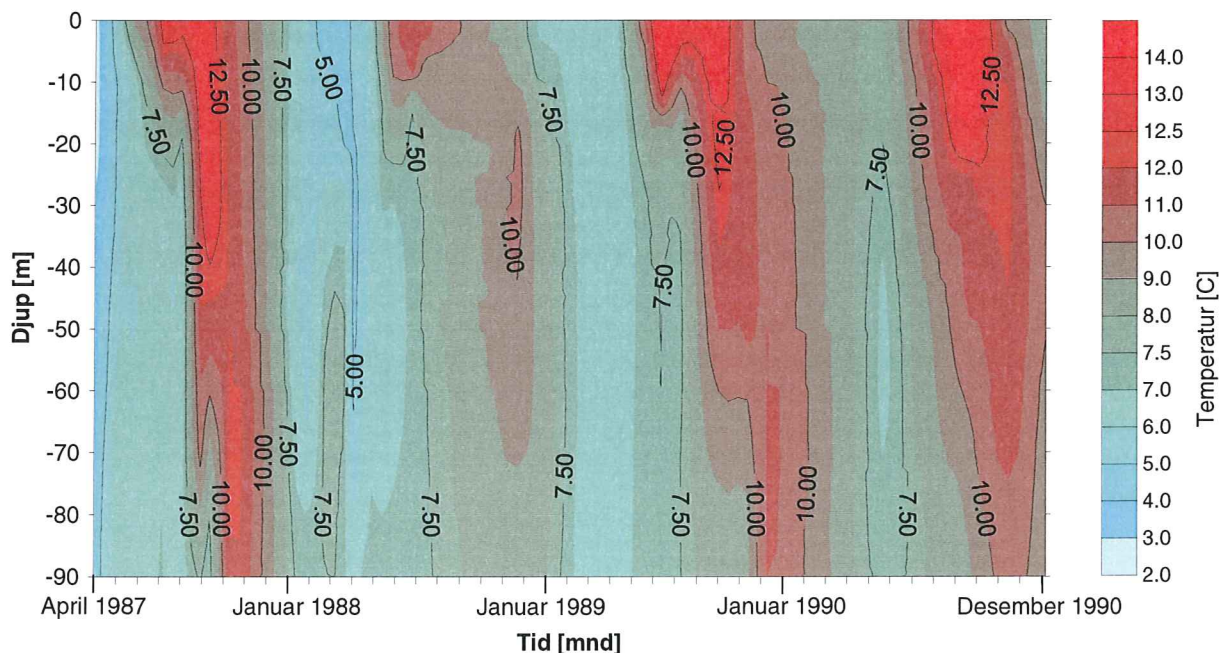
Figur 6. Isopletdiagram for sjøtemperatur målt av NIVA i perioden 1987-1990.
