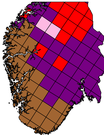
Figur 3 a) Dagens nitrogelekkasje. Beregnet etter data fra (Henriksen and Buan 2000). b) "Worst case" scenario for nitrogenlekkasje i 2010. Beregninger gjort med FAB-modellen med samme datagrunnlag som i figur a).
