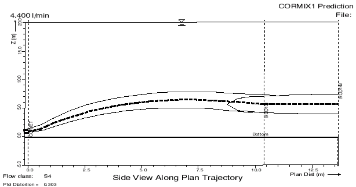
Figur 21. Tverrsnitt (X-Z) av utleppsskya i nærsonen fra utleppspunktet og nedstrøms til litt forbi innlagringspunktet i avstand ca 10 m.
