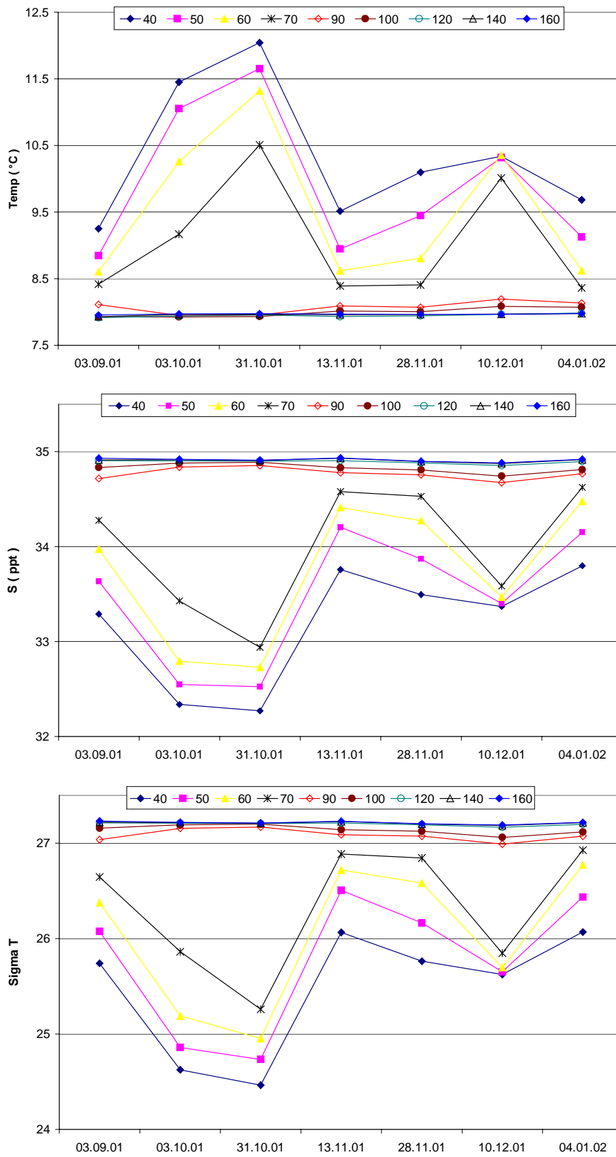
Figur 22. Tidsutvikling for temperatur, salinitet og sigma-t i ulike dyp fra 40 m og nedover til 160 m på Stasjon 2 (nær nytt sjøvassinntak), september 2001-januar 2002.
