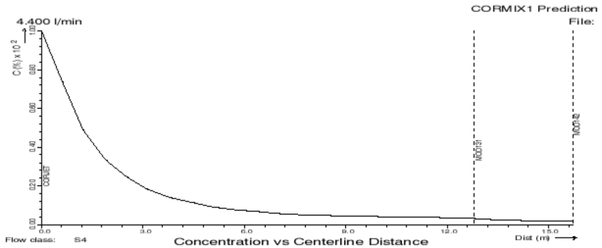
Figur 20. Simulert konsentrasjon nedstrøms utleppspunktet, for 15 cm/s strøm. Konsentrasjon i utleppsvatnet er vilkårlig satt lik 100. Innlagring som skjer i 10 m avstand fra utleppspunktet, motsvarer konsentrasjon på 100/28 = 3,6 . Sjå neste figur.
