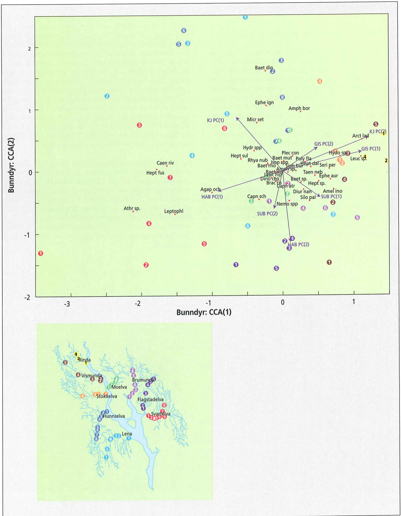
Figur 2.6.1 CCC analyse på binære bunndyrdata (EPT arter, til stedelikke tilstede) i forhold til ulike miljøparametre for mjoselvene.
