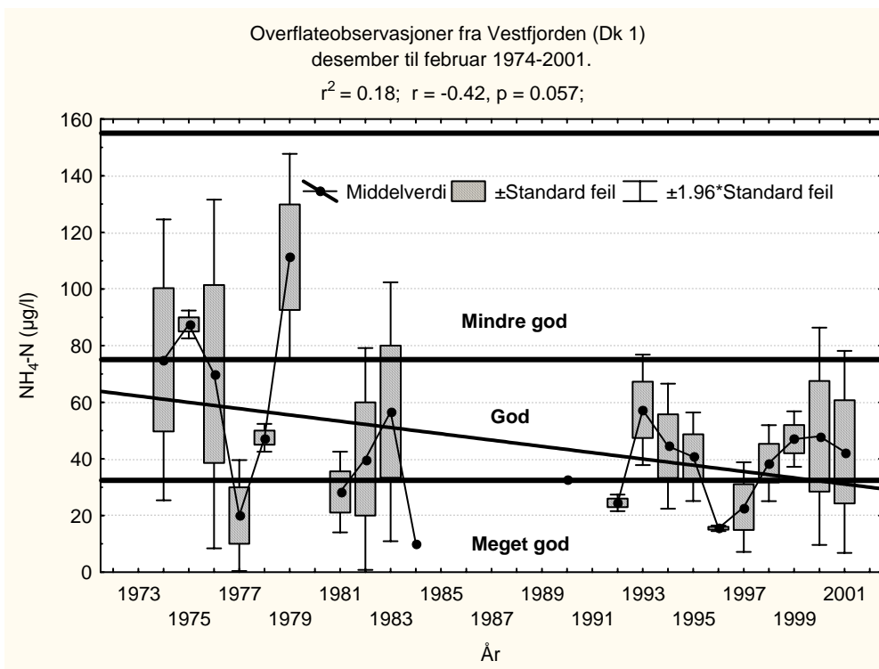
Figur 70. Overflateobservasjoner av ammonium i Vestfjorden (Dk 1), desember –februar 1974-2001. Vinterstid har konsentrasjonen ikke forandret seg signifikant. Sammenlignet med SFT's miljøklassifiseringsystem var tilstanden muligens noe dårligere på 1970-tallet. Dagens tilstand er god.
