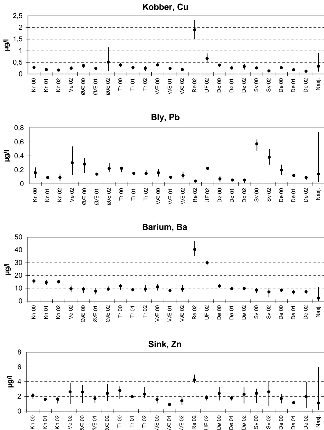
Figur 3. Konsentrasjoner av metaller i bekker og elver. Figuren viser middelværdier og variasjonsbredder de enkelte år. Kn = Knubba, Ve = Vesterengbekken, ØÆ = Østre Æra, Tr = Trøbekken, VÆ = Vestre Æra, Re = Rena ved Flåtestøa, UF = Utløp Flåtestøtjernet, Dø = Dønna, Sv = Svartbekken og De = Deia. Nasj. viser medianverdiene samt 10-prosentiler og 90-prosentiler fra en nasjonal undersøkelse av metaller i ferskvann (Skjelkvåle et al. 1996 og 1999).
