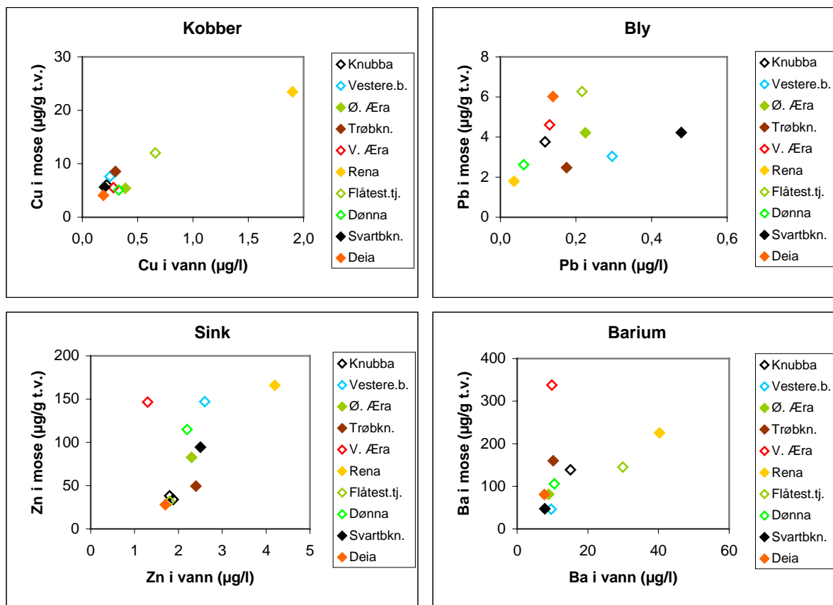
Figur 6. Sammenhengen mellom middelkonsentrasjoner av kobber (Cu), bly (Pb), sink (Zn) og barium (Ba) i vann og vannmose i bekker og elver med tilknytning til RØ.
