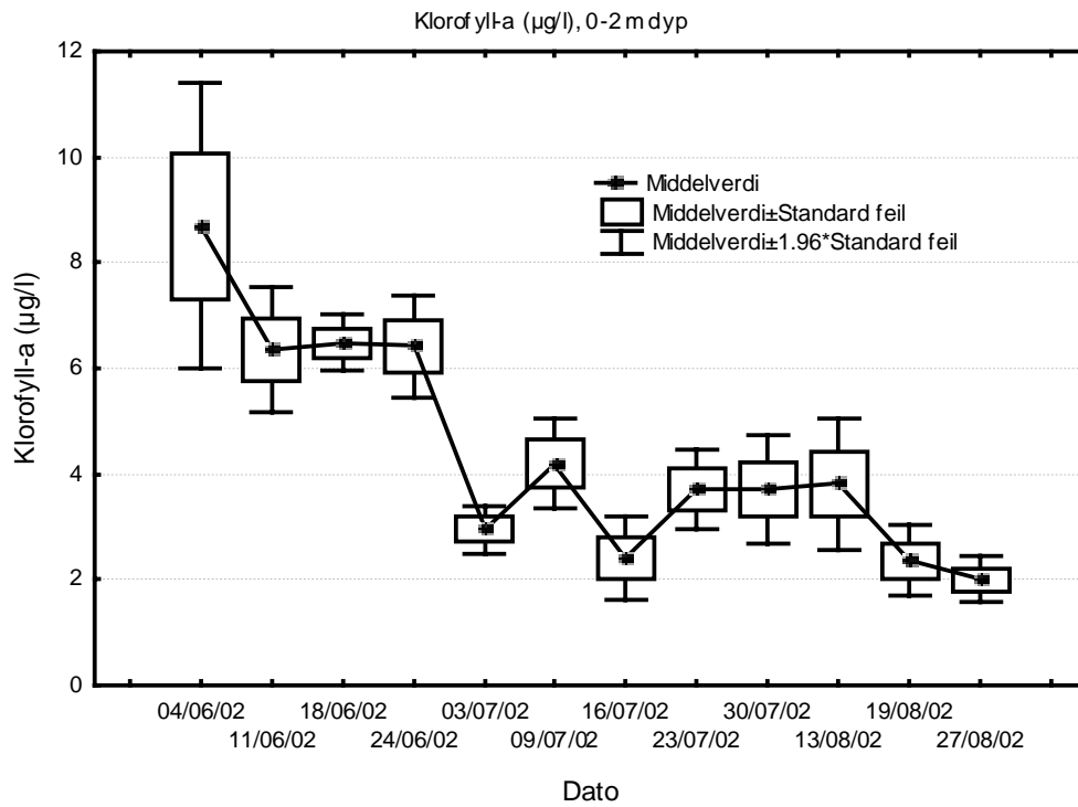
Figur 33. Klorofyll-a (µg/l) i 0-2 meters dyp, sommeren 2002. Middelvei av samtlige stasjoner. (Ukentlige observasjoner)
