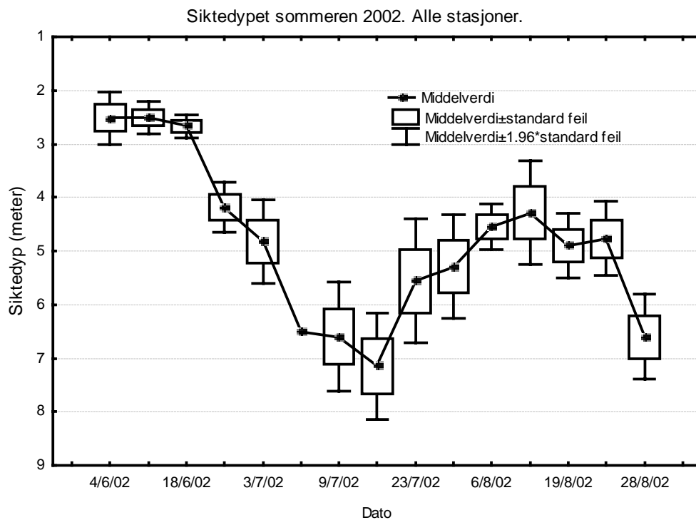
Figur 34. Siktedypet sommeren 2002. Middelvei av samtlige stasjoner. (Ukentlige observasjoner).
