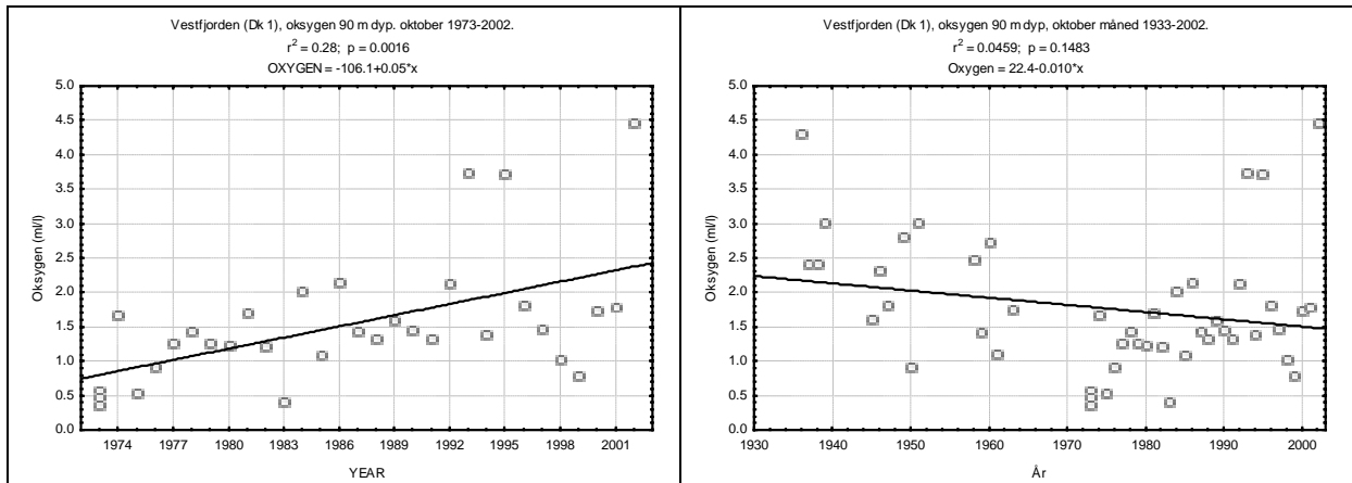
Figur 16. Oksygenkonsentrasjonen på 90 meter dyp (oktober måned) 1973-2002 og 1933-2002. Mens konsentrasjonen er signifikant økende 1973-2002 er den ikke (lengre) signifikant avtakende (som tidligere) mellom 1933-2002. De relativt store oksygenkonsentrasjonene i 1993, 1995 og 2002 bidrar til den positive utviklingen i 1973-2002, men sløyfes disse årene fra analysen vil den fortsatt være positiv. Derimot vil det bli en signifikant negativ trend i perioden 1933-2002.
