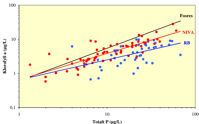
Figur 12. Sammenhengen mellom midlere algebiomasse (uttrykt som klorofyll a) og midlere fosformengde i innsjøer i Bergen 1992-2000. Hvert punkt angir sesongmiddel for en innsjø. Undersøkelser utført av Rådgivende Biologer er vist med blå punkter og regresjonslinje, mens undersøkelser utført av NIVA er vist i røde punkter og regresjonslinje. Til sammenligning er forventet sammenheng som uttrykt i Fosres-modellen (Berge 1987) vist som svart linje. Begge akser er logaritmiske.
