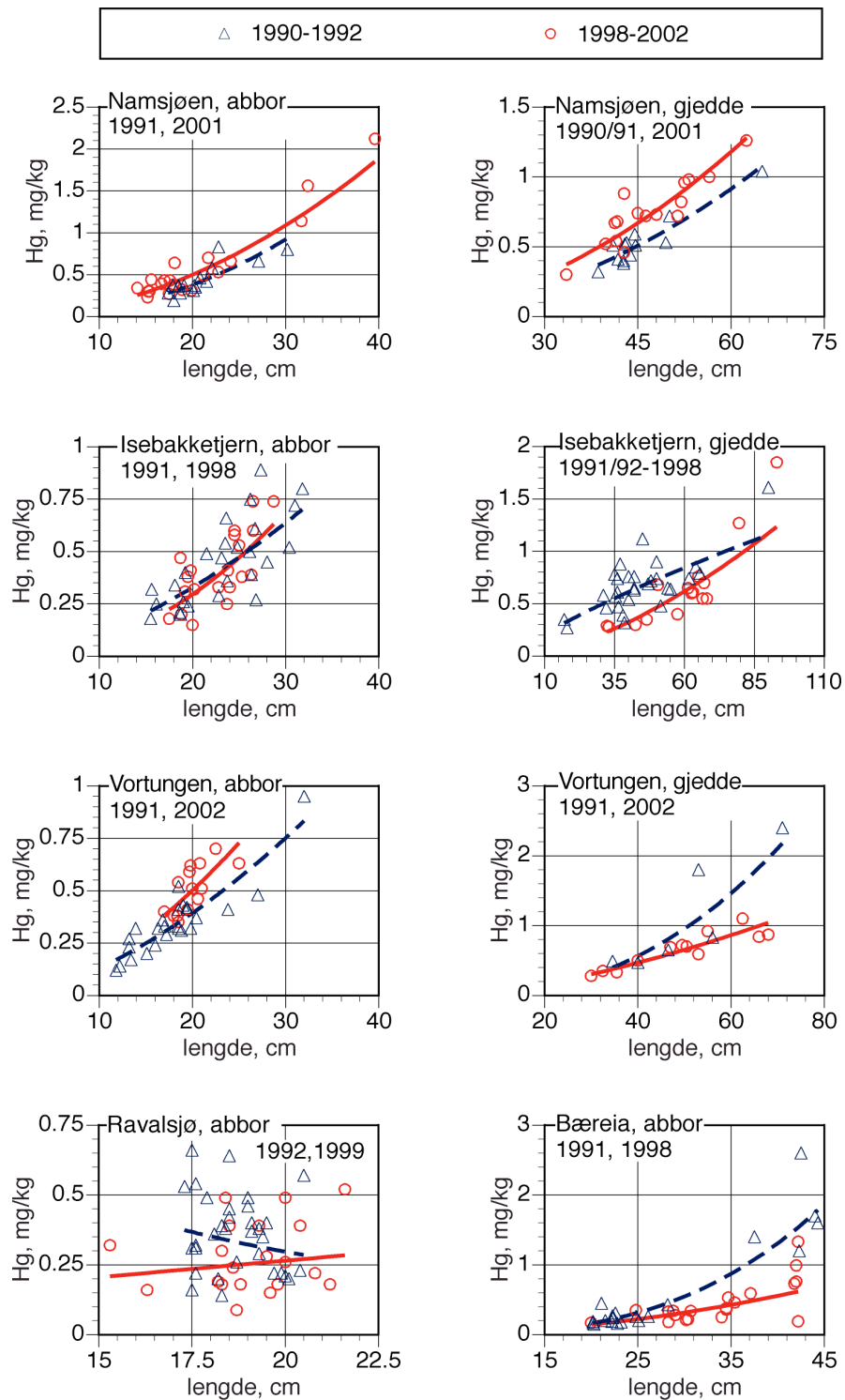
Figur 10. Kvikksølvkonsentrasjoner som funksjon av fiskelengde hos abbor og gjedde fanget i to tidsperioder (1990-1992 og 1998-2002). Kurvene er basert på lineære regresjoner av log-transformerte data.
