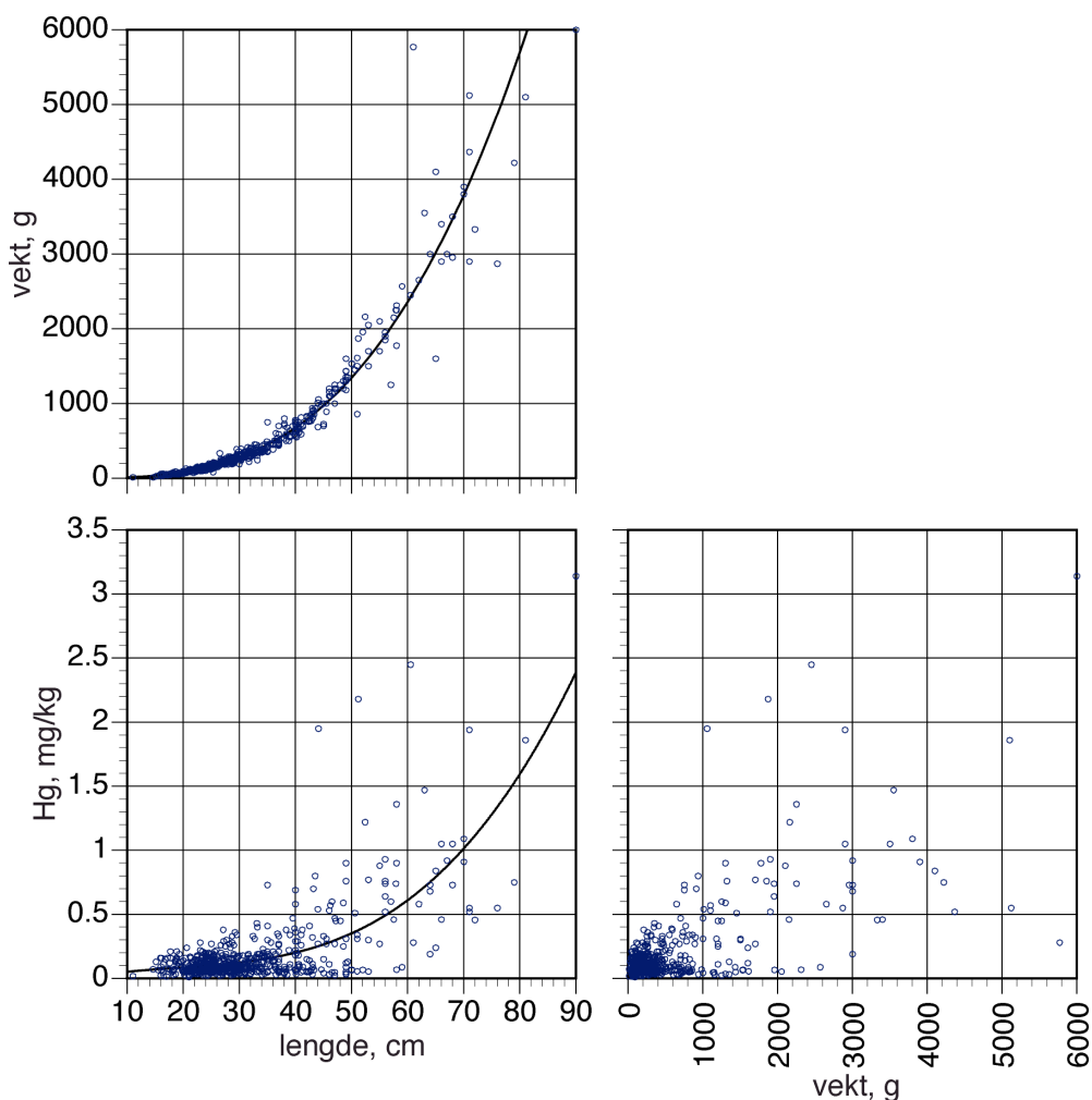
Figur 2. Sammenhengene mellom kvikksølvkonsentrasjon, lengde og vekt i ørret fra Sør- og Midt-Norge. Materialet er innsamlet i perioden 1999-2002. Antall bestander: 38, antall fisk: 623.
