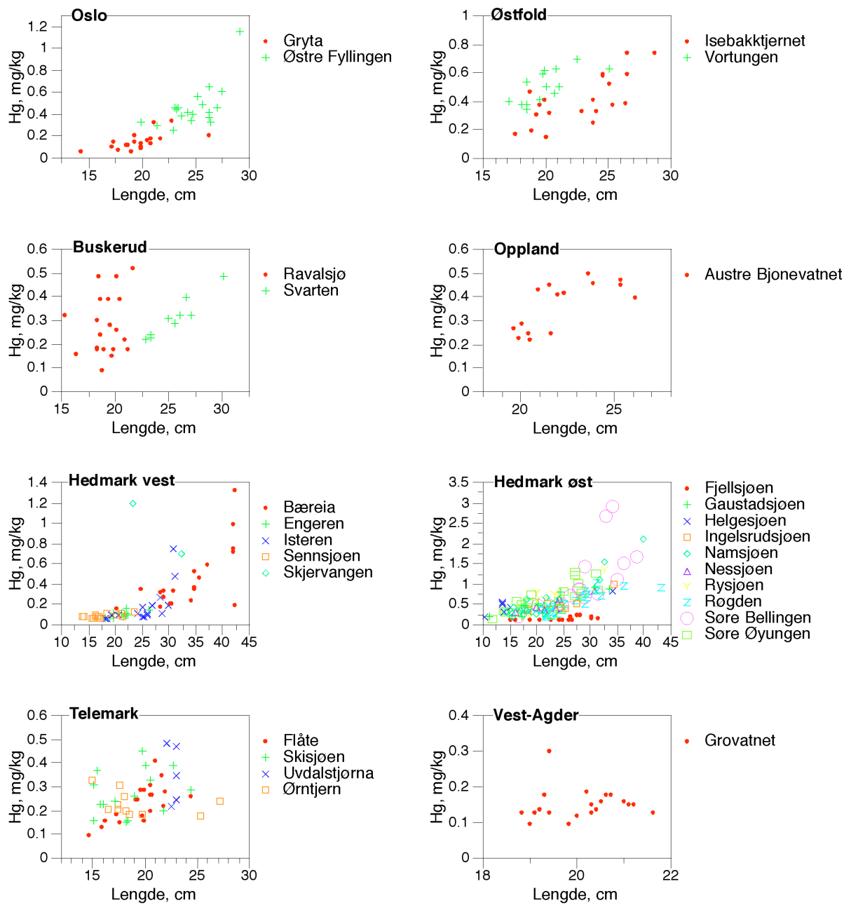
Figur 5. Kvikksølv i abbor, konsentrasjoner plottet mot fiskelengde. De enkelte bestandene er gruppert fylkesvis. Hedmark vest og øst er henholdsvis innen UTM sone 32 og 33. Fangstår: 1999–2002. Antall bestander: 27. Antall fisk: 409.
