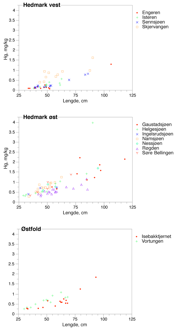
Figur 7. Kvikksølv i gjedde, konsentrasjoner plottet mot fiskelengde. De ulike bestandene er gruppert fylkesvis. Hedmark vest og øst er henholdsvis innen UTM sone 32 og 33. Fangstår: 1999–2002. Antall bestander: 13. Antall fisk: 137.
