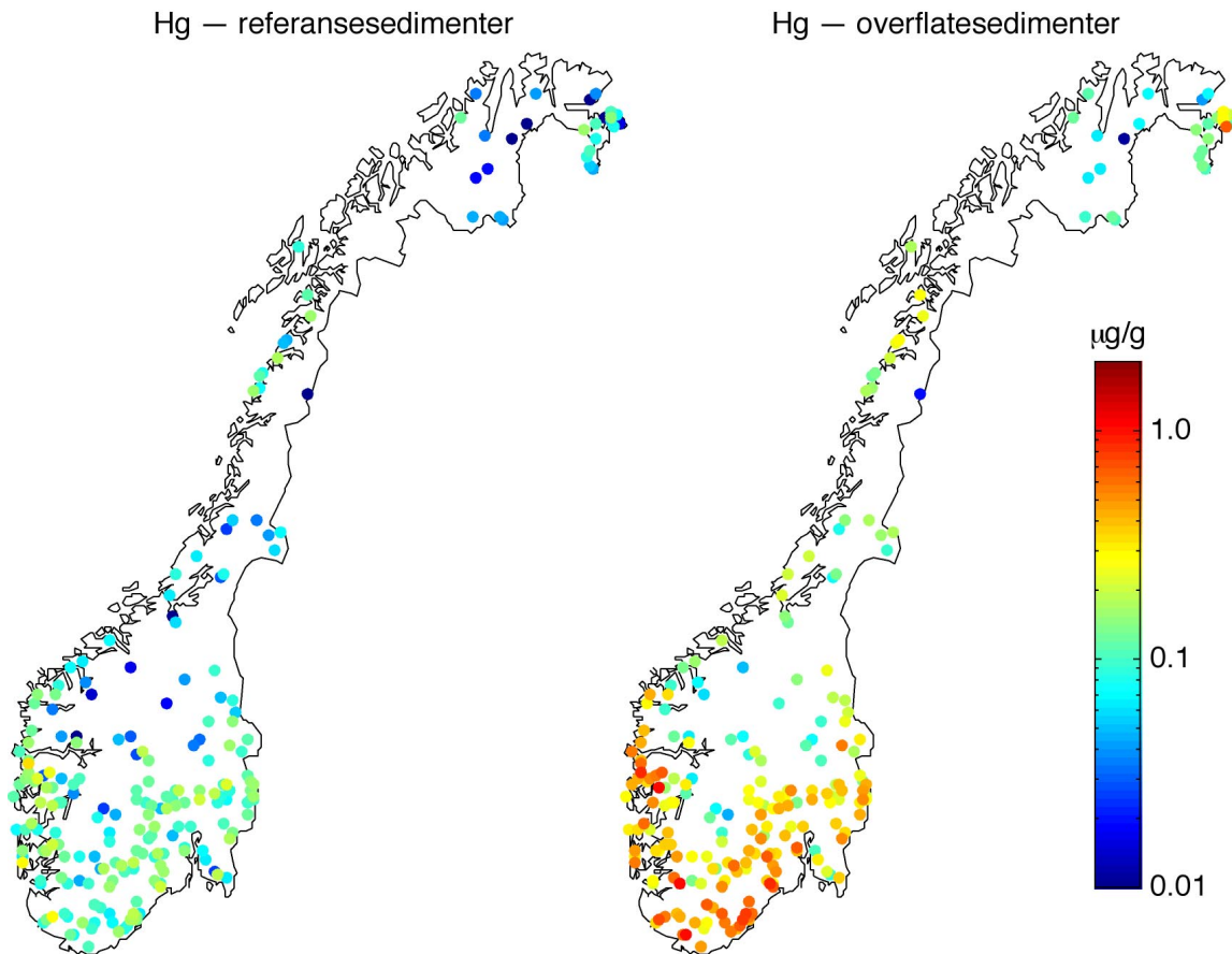
Figur 1. Kvikksølvkonsentrasjonen i norske innsjøsedimenter. Overflatesedimentene er fra det øvre 0,5 cm sjiktet, referansesedimentene er førindustrielle sedimenter (2 cm tykt sjikt, 30–50 cm under sediment-overflaten). Konsentrasjonsøkningen skyldes i all hovedsak avsetninger av atmosfæriske forurensninger. Innsjøene ( n = 231 ) ble prøvetatt i 1995-96. Figuren er fra Rognerud et al. (1999).
