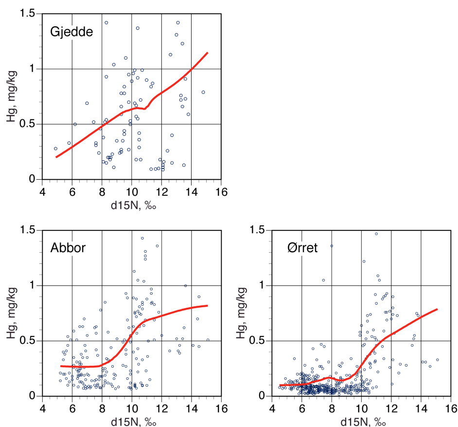
Figur 8. Sammenhengen mellom kvikksølvkonsentrasjon og stabile N-isotoper ( \delta^{15}\text{N} ). Isotopforholdet kan benyttes som et mål på fiskens trofisk nivå (plass i næringskjeden). Kurvene er basert på en estimator fra en lokalt vektet regresjonsmodell (LOWESS), som er i stand til å fange opp ulineære kurveforløp. Ørret: 27 bestander, 445 individer. Abbor: 16 bestander, 203 individer. Gjerdde: 11 bestander, 90 individer.
