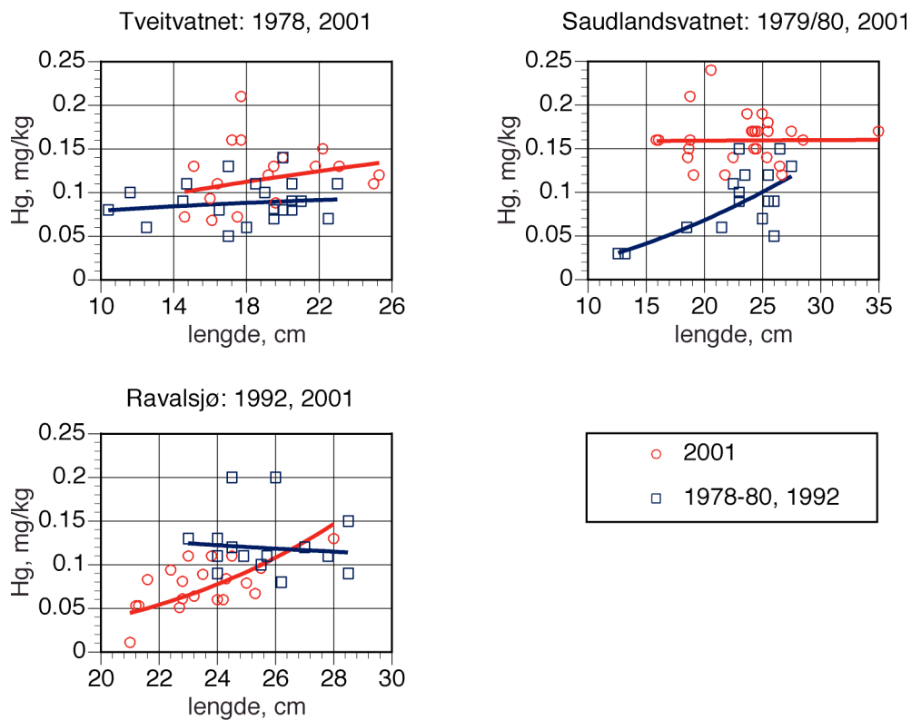
Figur 9. Kvikksølvkonsentrasjoner som funksjon av fiskelengde hos ørret fanget i periodene 1978-80/1992 og i 2001. Kurvene er basert på lineære regresjoner av log-transformerte data.
