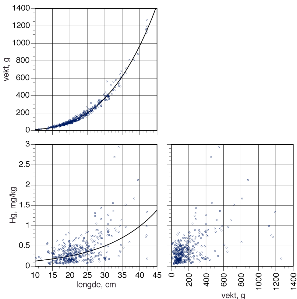
Figur 4. Sammenhengene mellom kvikksølvkonsentrasjon, lengde og vekt i abbor fra Sør-Norge. Materialet er innsamlet i perioden 1999-2002. Antall bestander: 26, antall fisk: 407.
