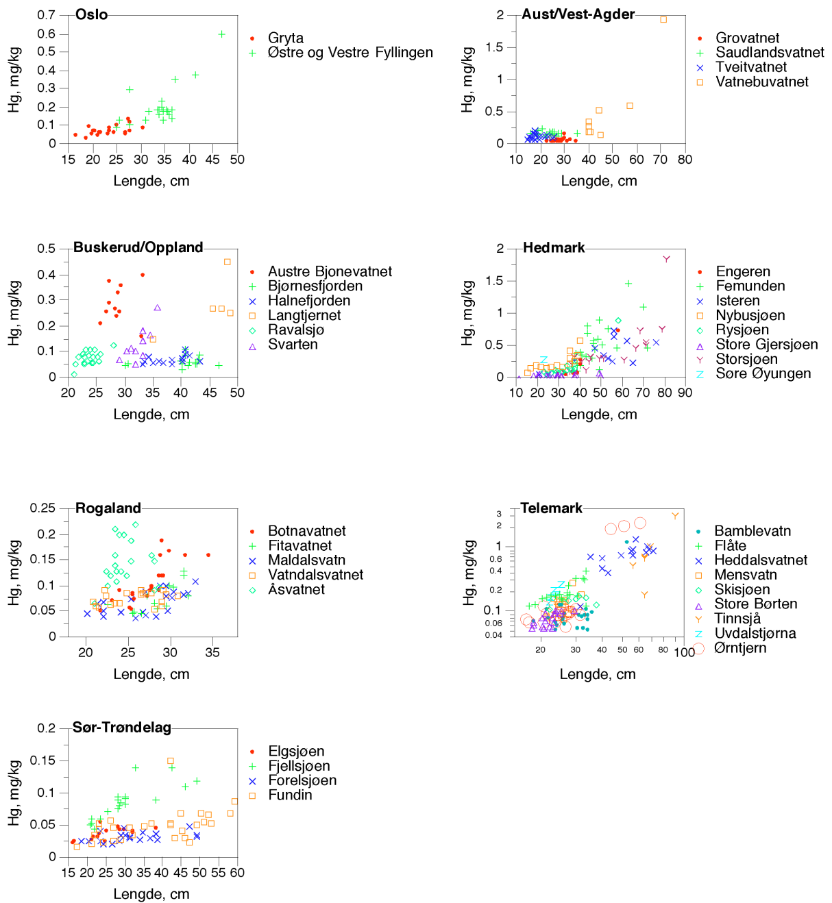
Figur 3. Kvikksølv i ørret, konsentrasjoner plottet mot fiskelengde. De ulike bestandene er gruppert fylkesvis. Fangstår: 1999–2003. Antall bestander: 38. Antall fisk: 623.
