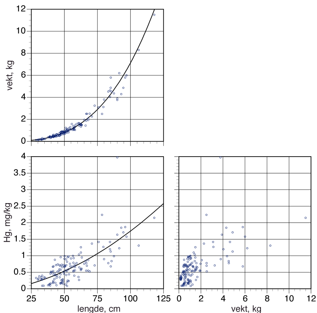
Figur 6. Sammenhengene mellom kvikksølvkonsentrasjon, lengde og vekt i gjedde fra Øst-Norge. Materialet er innsamlet i perioden 1998-2001. Antall bestander: 13, antall fisk: 137.
