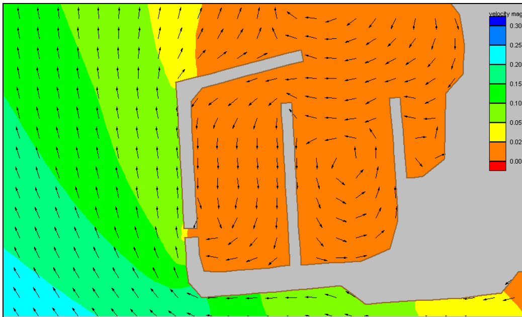
Figur 8. Scenario 3a: Strømbilde for 0-2 m vannlag med ny betongmolo, kulvert (ca. 3 m bred) og ved nordgående strøm. Topografien er litt forskjellig fra Fig. 4-5, uten at det har noen betydning for resultatene.
