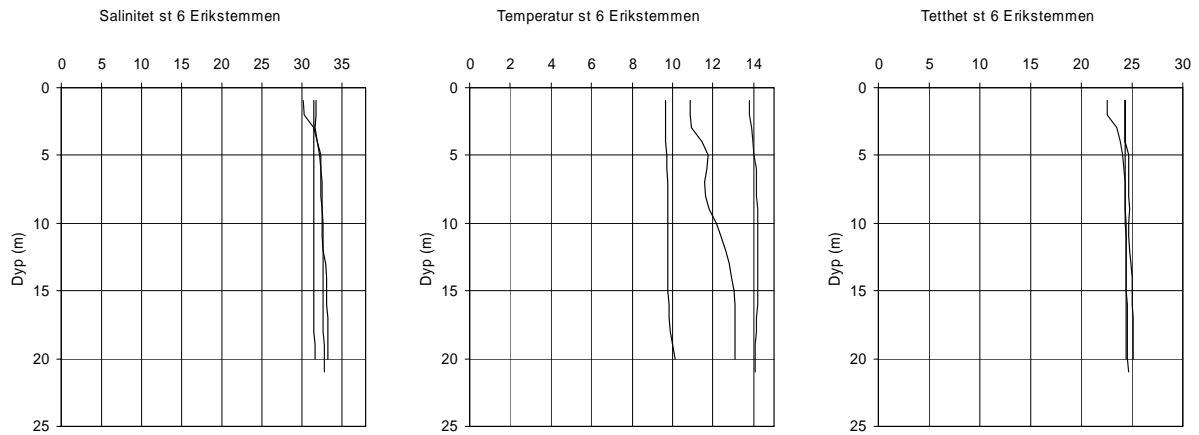
Figur 7. Profiler for saltholdighet, temperatur og tetthet i Stolsfjorden ved utslippet fra Erikstemmen avfallsplass målt med CTD-sonde høsten 2003 (1. okt – 12. nov).
