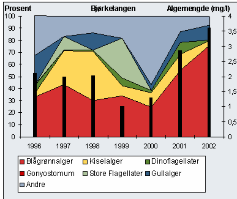
Figur 4. Algemengde og sammensetning av algesamfunnet i Bjørkelangen. Søylene gir algemengden i mg/l (høyre skala), mens den fargede bakgrunnen gir sammensetningen av de viktigste hovedgruppene i prosent. (fra Fylkesmannen i Akershus sine hjemmesider).
