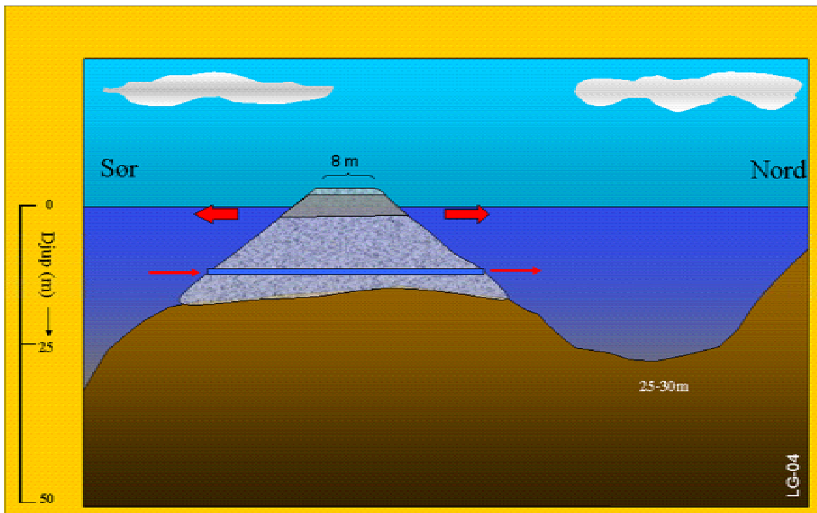
Figur 26. Omtrentleg skisse av tverrsnitt av fylling i hovedsundet mellom Litle og Store Bukken. Med kulvert (seglingsopning) og gjennomstrømningsrør.
