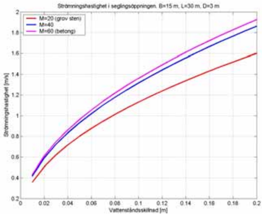
Figur 30. Strømfart i seglingsoppninga som funksjon av skilnad i vassstand frå sør-til nordside av fyllinga (t.d. som følgje av vindoppstuving). Kurvene er basert på tre ulike Mannings tal ( M ), som svarar til ulikt materiale med friksjon.
