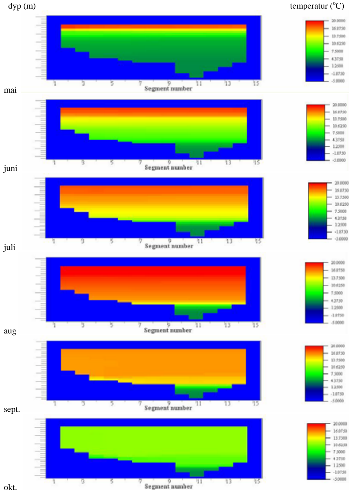
Figur 10. Simulert temperatur i Aurevann 2004.
