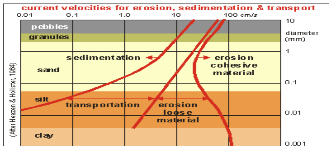
Figur 13. Sammenheng mellom erosjon av sedimenter (vist som kornstørrelse) og strømhastighet.
