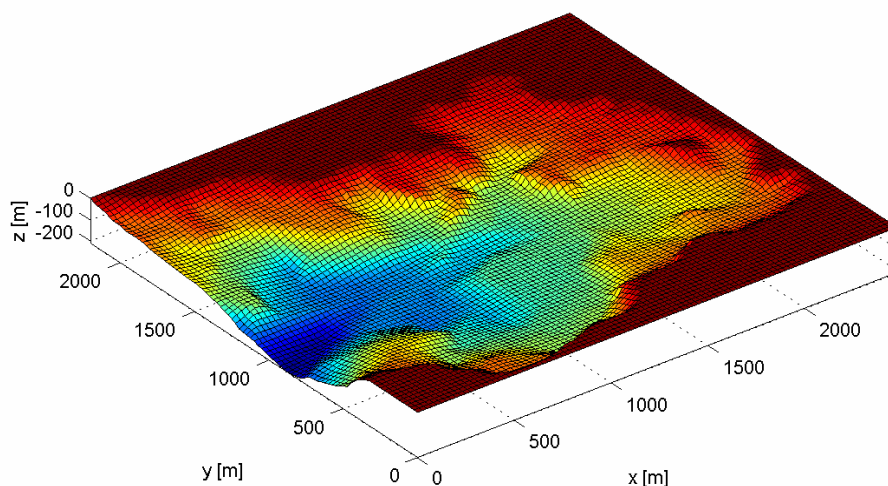
Figur A1. Numerisk nett (grid) for de todimensjonale strømmodellingene med RMA2. Nettet har 25 meters oppløsning og 100 x 89 noder.
