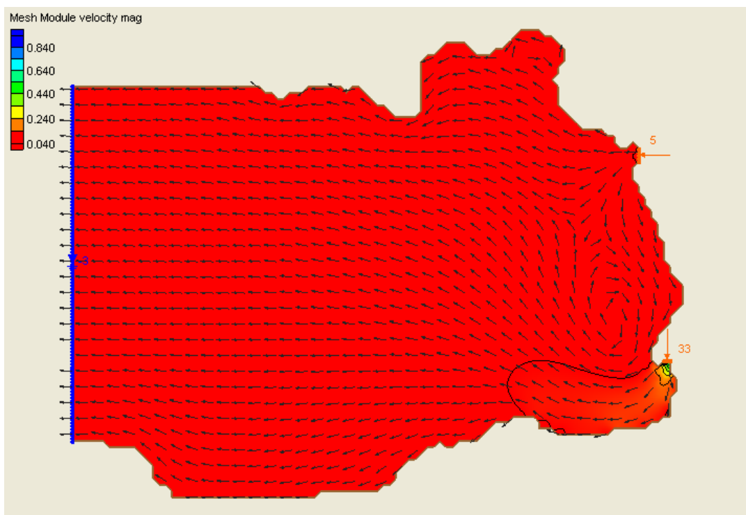
Figur 15. Resultat fra RMA2-modelleringene med flat bunn (konstant dyp 2 m). Modellen drives av ferskvanntilførsel 33 \text{ m}^3/\text{s} fra Sauda III og 5 \text{ m}^3/\text{s} fra Nordelva/Storelva.
