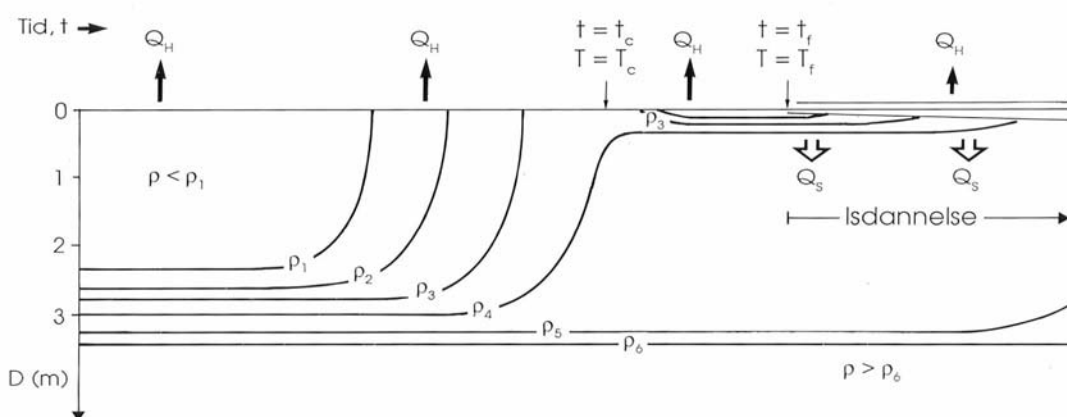
Figur 11. Tidsforløpet for konveksjon i overflatelaget og dannelse av is under avkjøling.
