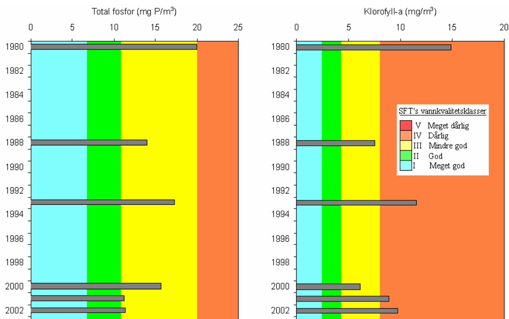
Figur 5. Eutrofisituasjonen i Jarenvatnet gitt som hhv. midlere fosforkonsentrasjon og midlere algemengde (klorofyll-a) i sommerhalvåret for de år vi har data fra. Tallene viser ingen signifikant bedring i eutrofi-situasjonen etter 1988.
