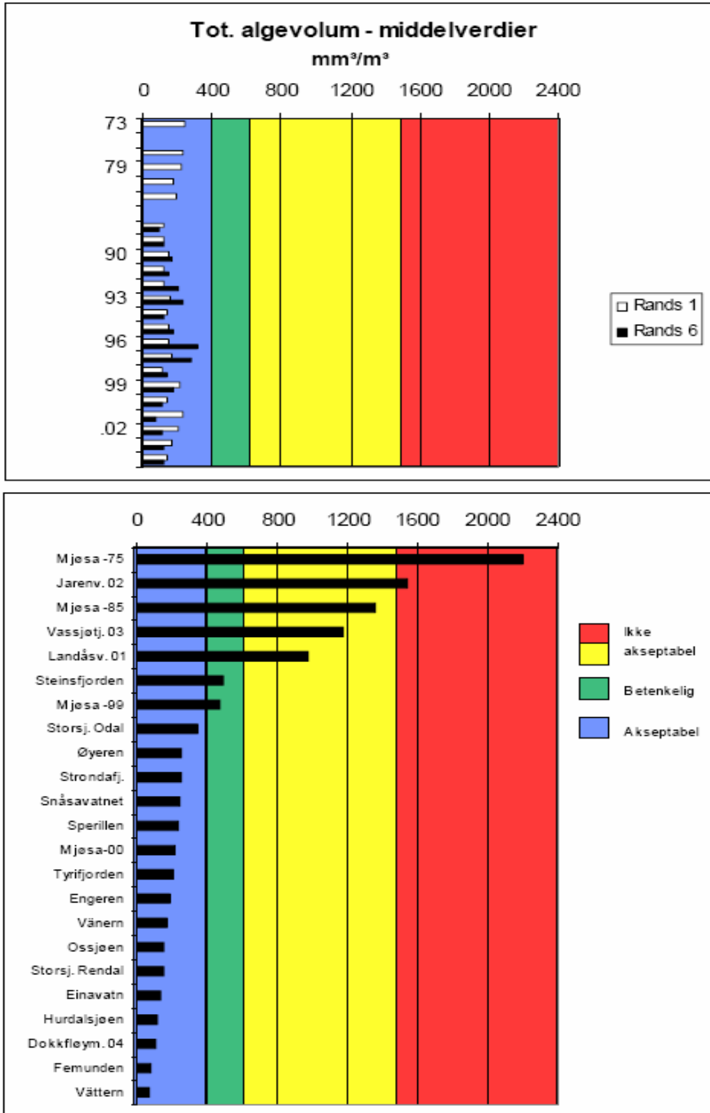
Figur 6. Algemengde (mm 3 /m 3 ) i Randsfjorden i ulike år (øvre panel), sammenliknet med Jarenvatnet 2002 og en del andre innsjøer (nedre panel). (etter Løvik, Kjellberg og Brettum 2005).
