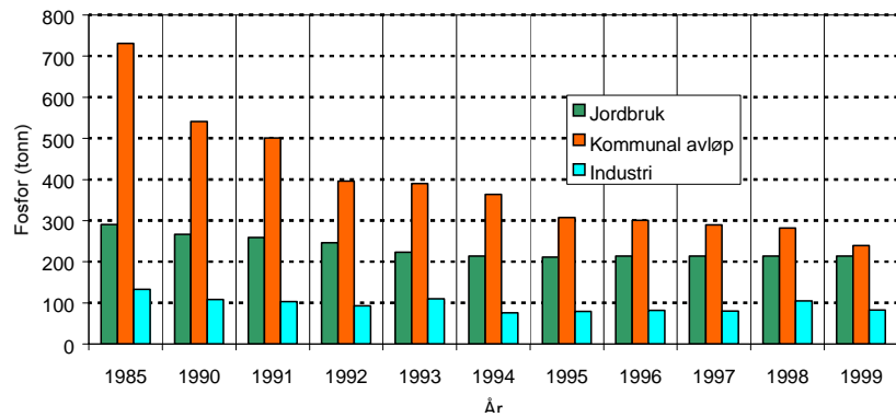
Figur 4. Beregnede norske tilførsler av fosfor (tot-P) fra jordbruk, kommunalt avløp og industri fra 1985 og 1990-99 til Skagerrakkysten (svensegrensen-Lindesnes) (Borgvang og Tjomsland, 2001)(fra Moy et al.) 2002).
