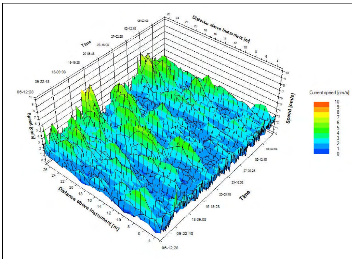
Figur 10. 3-dimensjonalt bilde som viser strømhastigheten fra ca.30 m dyp og opp til ca. 7 m dyp som funksjon av tiden. I alt vesentlig er hastigheten mindre enn 7 cm/s.
