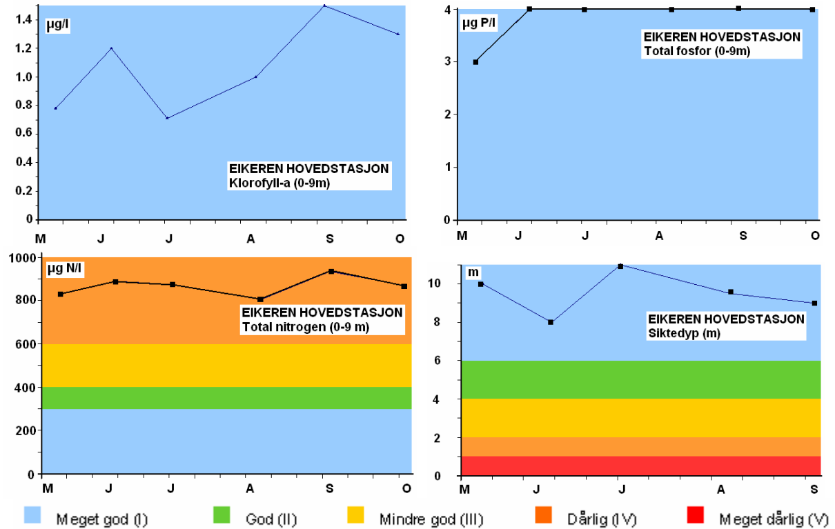
Figur 2. Resultater fra Hovedstasjonen i Eikeren ut for Tryterød i 2005
