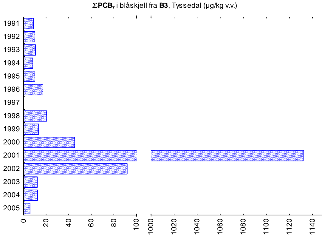
Figur 14. \Sigma\text{PCB}_7 i blåskjell fra Tyssedal (st. B3; 1991-2005), \mu\text{g/kg} våtvekt. Verdiene er også gjengitt i Tabell 12. (| = høyt bakgrunnsnivå). Mrk. brudd på aksen mellom 100 og 1000.
