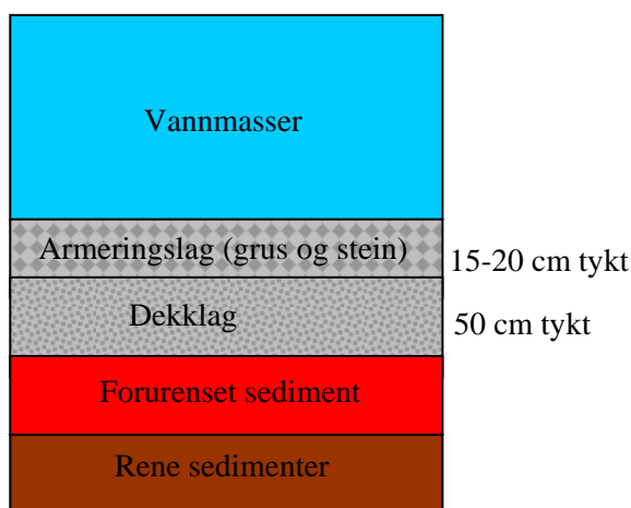
Figur 27.. Utforming av tildekkingslaget.
