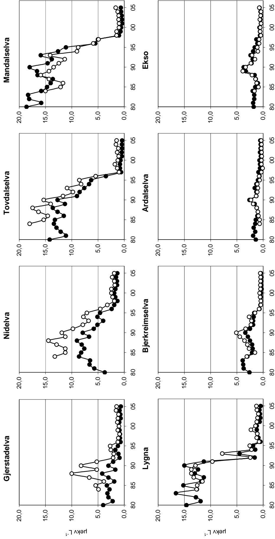
Figur 33. H^+ og labilt Al i kalka elver. H^+ ● og labilt Al ○. Enhet: \mu\text{ekv L}^{-1} .
