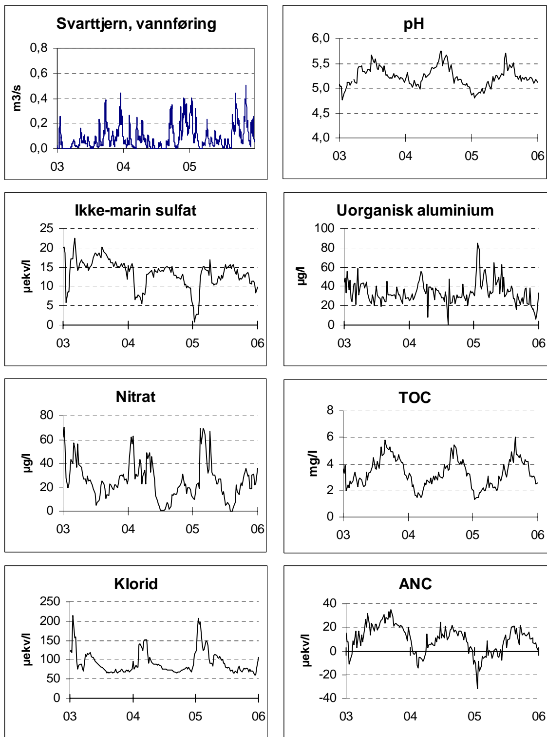
Figur 16. Variasjon i avrenning og konsentrasjon for en del forskjellige kjemiske parametre i Svartetjern 2003 - 2005.
