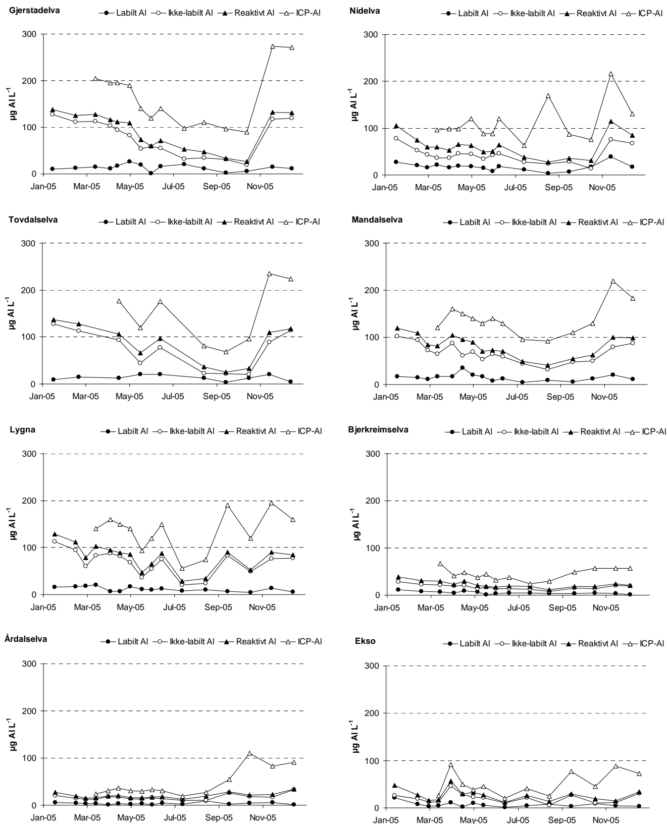
Figur 37. Sesongmessig fordeling av ulike aluminiumsfraksjoner i de kalkdede elvene i 2005. ICP-Al er synonymt med totalt aluminium.
