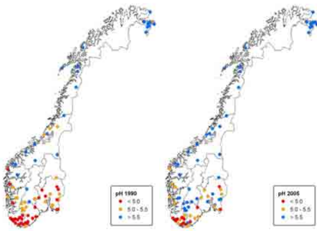
Figur 18. pH i overvåkingsinnsjøene i 1990 og 2005. Figuren illustrerer tydelig forbedringen i forurensingssituasjonen.
