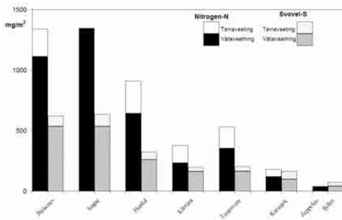
Figur 6. Estimert totalavsetning (sum av våt- og tørravsetning) av svovel- og nitrogenforbindelser på norske bakgrunnsstasjoner i 2005.
