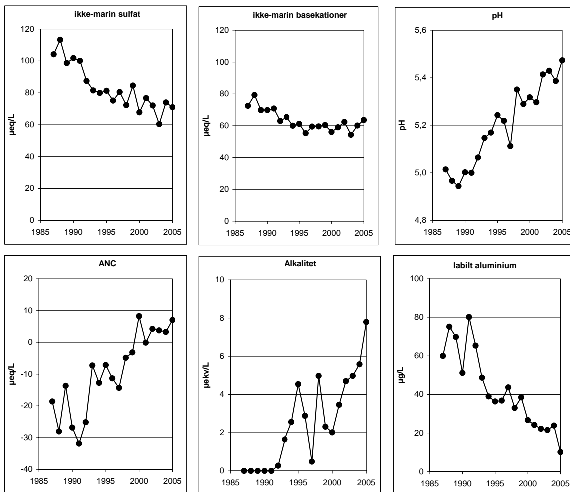
Figur 29. Forsuringsparametre for seks småvann på Jarfjordfjellet i 1987-2005. Middelerverdier for basekationer, sulfat ( SO_4^* ), ANC, alkalitet, pH og labilt aluminium.
