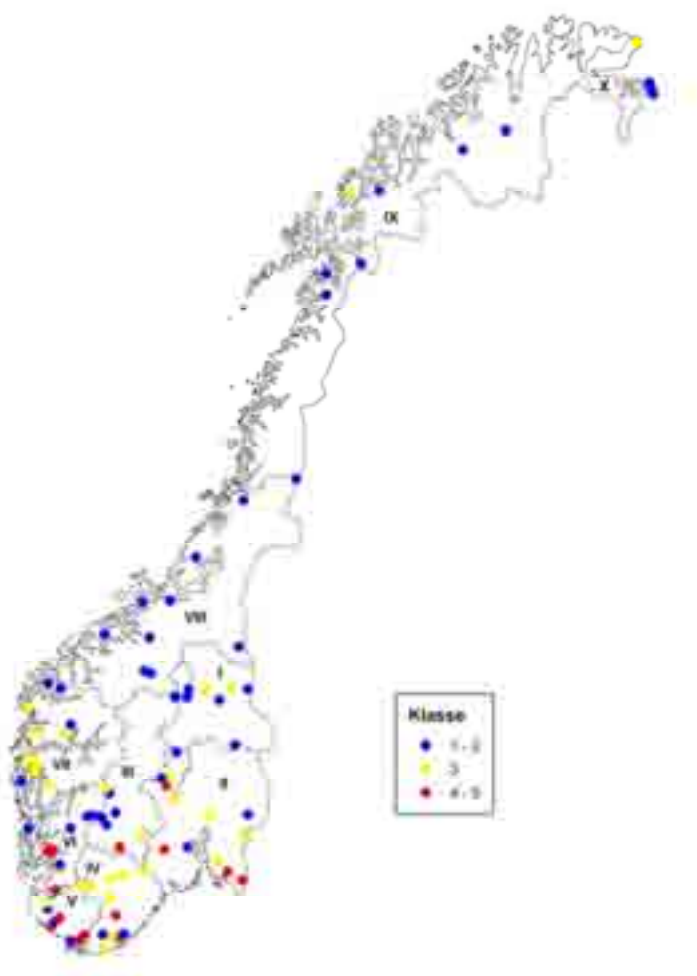
Figur 50. Kart med angivelse av forsuringskader basert på bunndyr og planktoniske og litorale krepsdyr (innsjøer) fra siste undersøkelses år. Klasse 1-2: ingen/ubetydelig til litt forsuringskadet, klasse 3: moderat forsuringskadet, klasse 4-5: sterkt til svært sterkt forsuringskadet.
