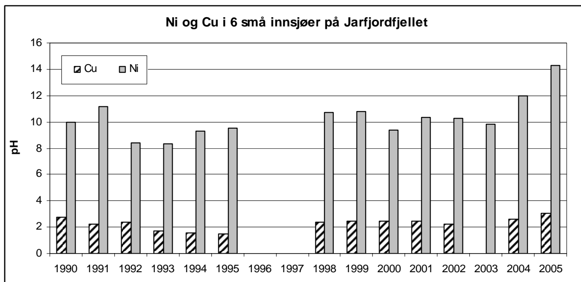
Figur 30. Årlige middelerverdier for nikkell og kobber i seks små innsjøer på Jarfjordfjellet fra 1990 til 2005).
