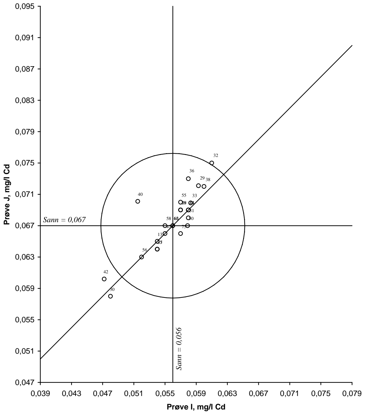
Figur 25. Youndendiagram for kadmium, prøvepar IJ Akseptansegrensen, angitt med en sirkel, er 15 %
