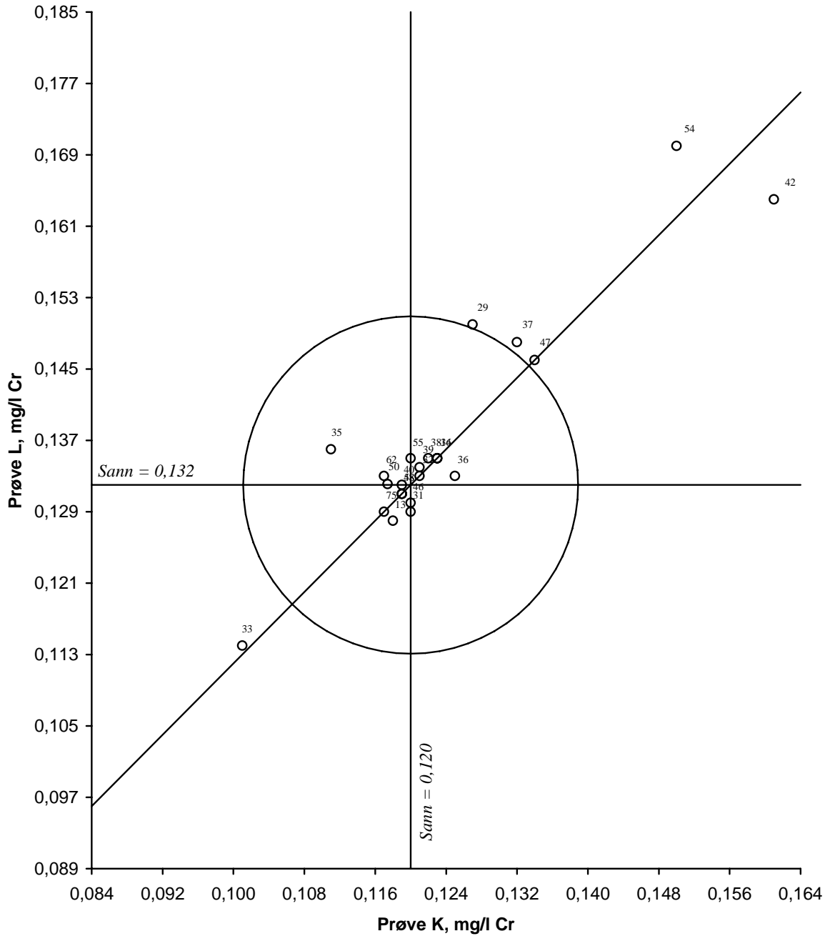
Figur 30. Youdendigram for krom, prøvepar KL Akseptansegrensen, angitt med en sirkel, er 15 %
