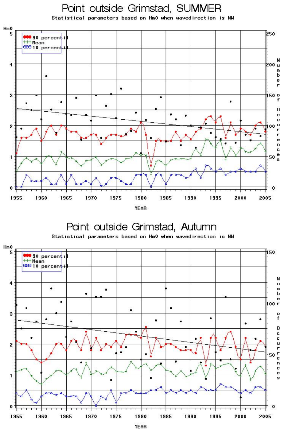
Figur A.5.14. Statistiske parametere basert på Hm0 (signifkant bølgehøyde) når bølgeretningen er fra NW sommerstid (ovre panel) og om høsten (nedre panel) ved Grimstad.
