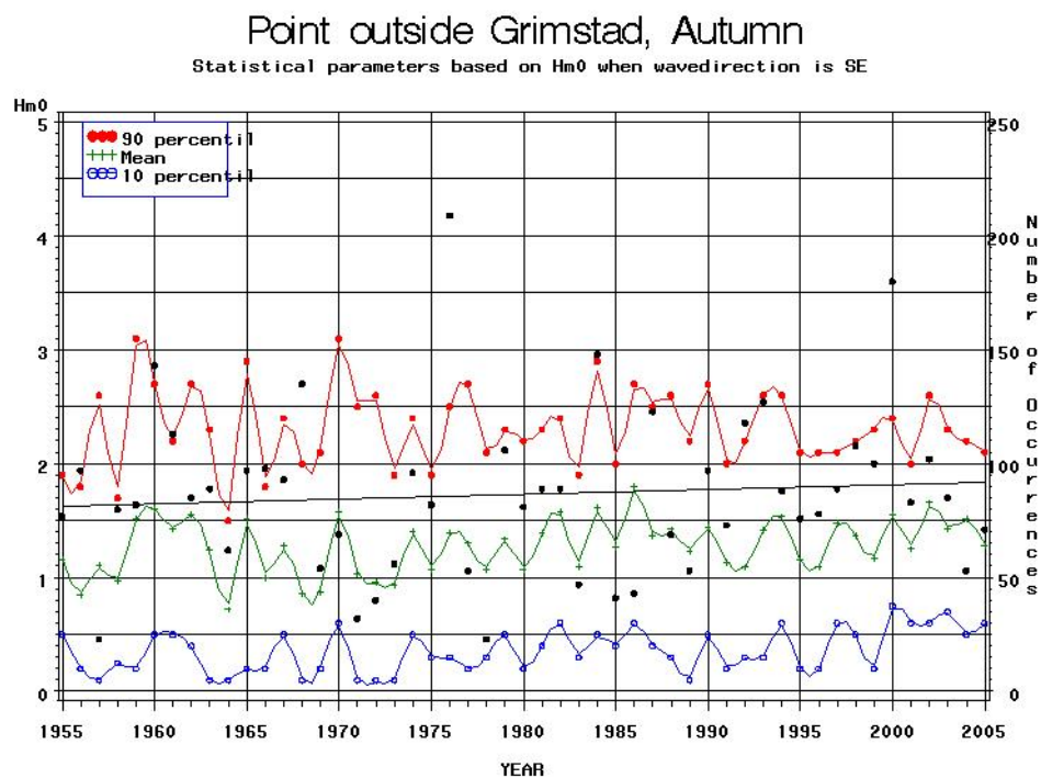
Figur A.5.18. Statistiske parametere basert på Hm0 (signifikant bølgehøyde) når bølgeretningen er fra SE sommerstid (ovre panel) og om høsten (nedre panel) ved Grimstad.
